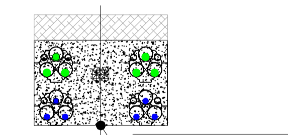
DETAIL 1: HIGH VOLTAGE TRENCH UNDER LAND AREA (2x132kV + 2x132kV CABLES) / DETALLE 1: ZANÍA LÍNEA ALTA TENSIÓN BAJO TERRENO (2X132KV + 2X132KV CABLES)
