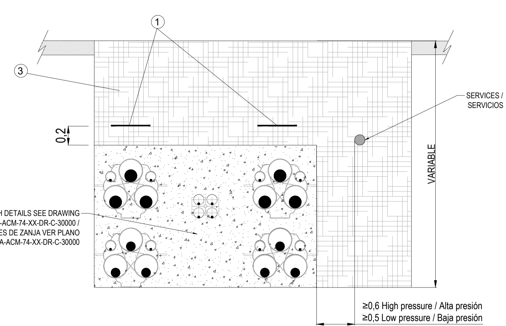
DETAIL 3: TYPICAL SECTION FOR PARALLEL SERVICES (GAS PIPELINES) SECCIÓN TÍPICA PARA SERVICIOS PARALELOS (TUBERÍAS DE GAS)
