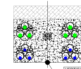
DETAIL 1: HIGH VOLTAGE TRENCH UNDER LAND AREA (2x220kV + 2x132kV CABLES) / DETALLE 1: ZANJA LÍNEA ALTA TENSIÓN BAJO TERRENO (2x220kV + 2x132kV CABLES)
