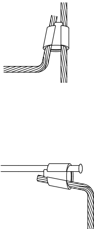
CONECTORES AMPACT PARA ENLACES Cu/Cu Y Cu/PICA EN PUESTA A TIERRA
