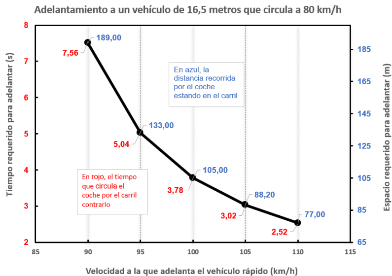
Figura 6.11: Reducción de tiempo y espacio de adelantamiento con el aumento de la velocidad (elaboración propia).
