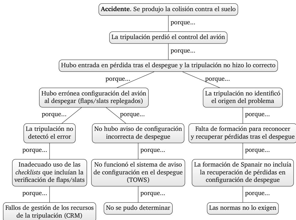
Figura 5.7: Identificación de causas en el accidente de Spanair del año 2008. Cada bloque se puede interpretar como un síntoma, o una consecuencia, del hecho recogido en el bloque siguiente (elaboración propia).
