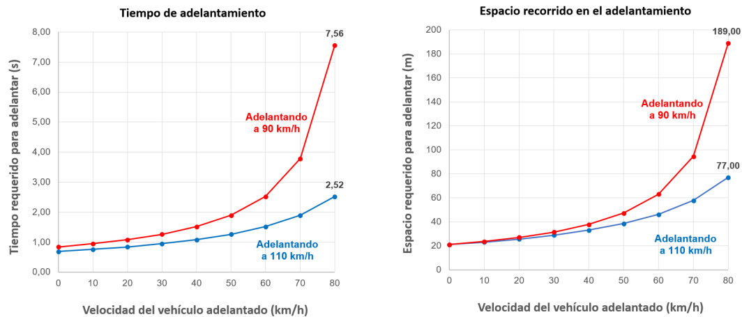
Figura 6.10: Comparativa de tiempos y espacios de adelantamiento (elaboración propia).
