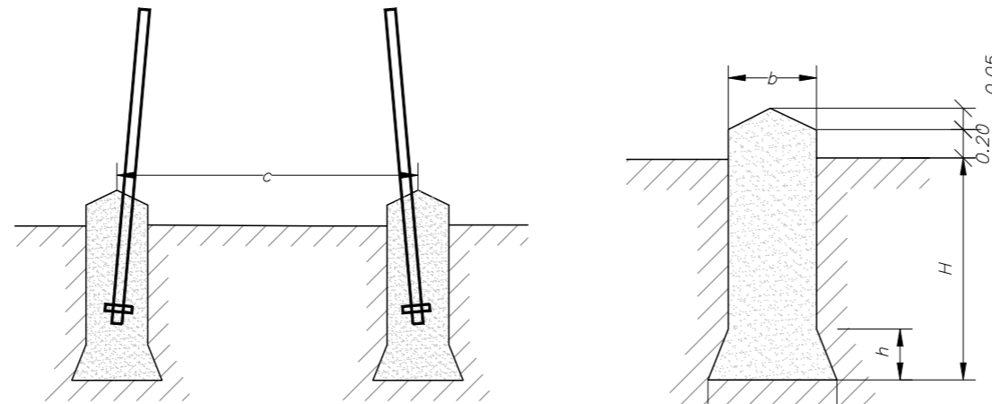
CIMENTACIÓN TETRABLOQUE (Cuadrada con cueva)
