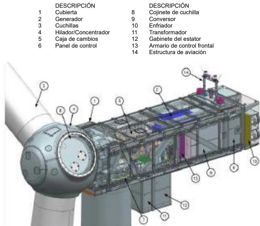
Imagen 5. Representación 3D componentes aerogenerador.
