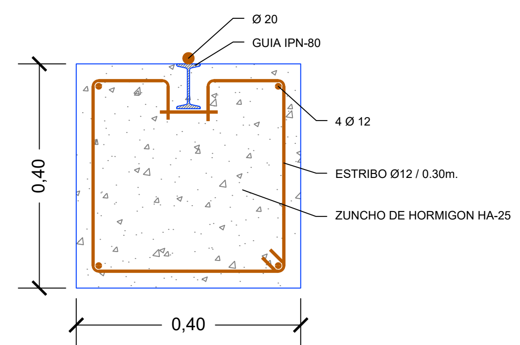
DETALLE 1
