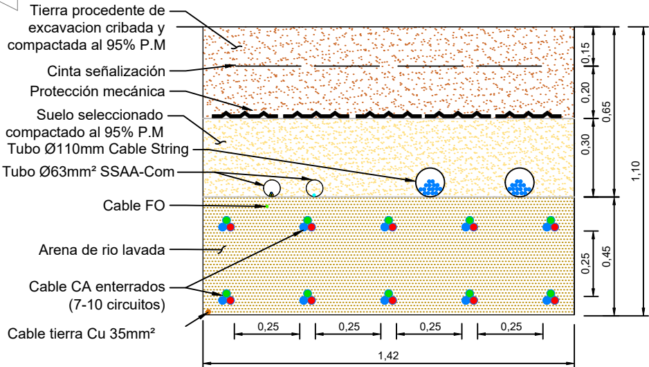
TIPO BT9-10C
