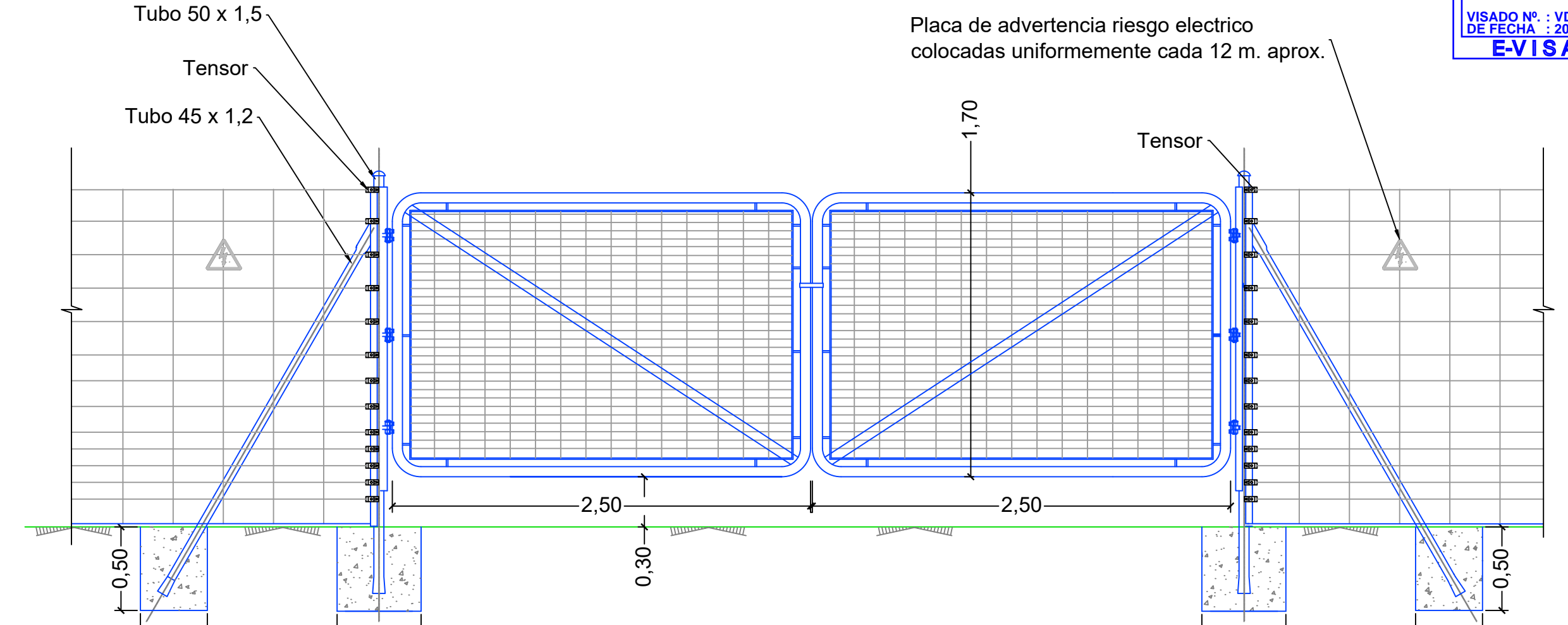
PUERTA PROVISIONAL
