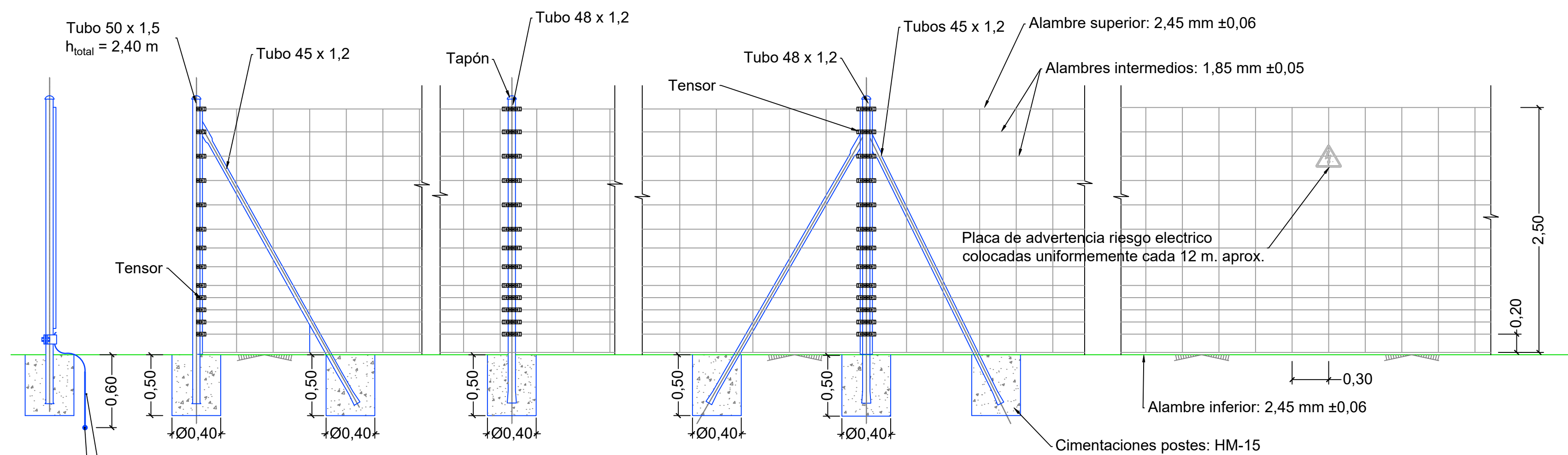
ALZADO
