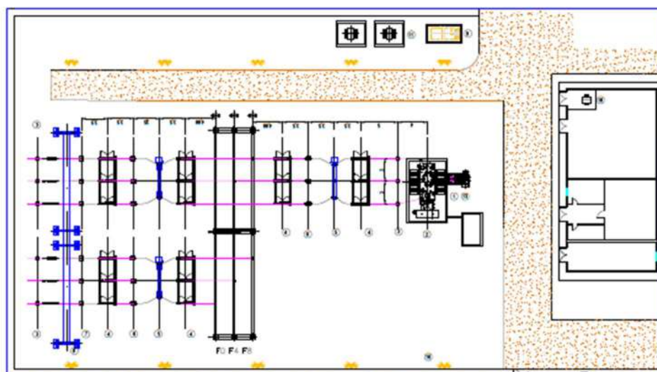
Ilustración 13. Planta SET
