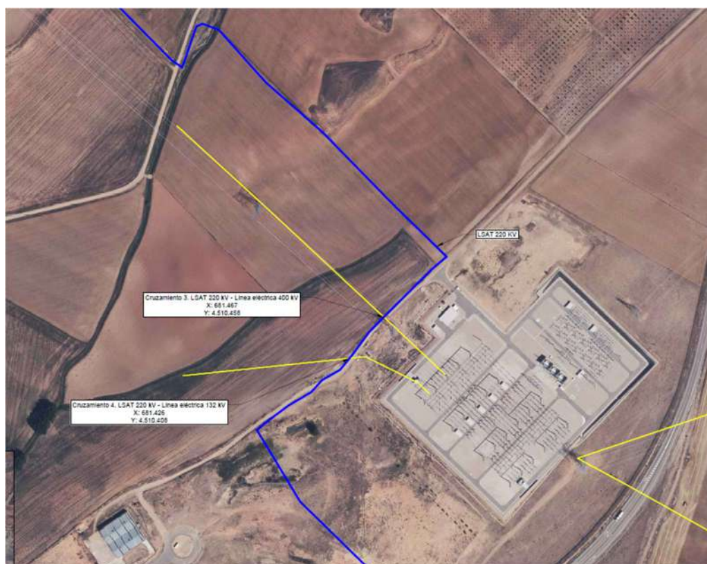
Ilustración 25. Afección a líneas eléctricas (3/3)
