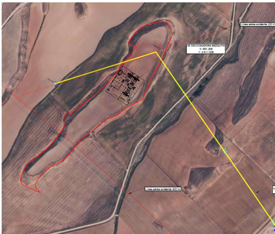
Ilustración 26. Afección a líneas eléctricas
