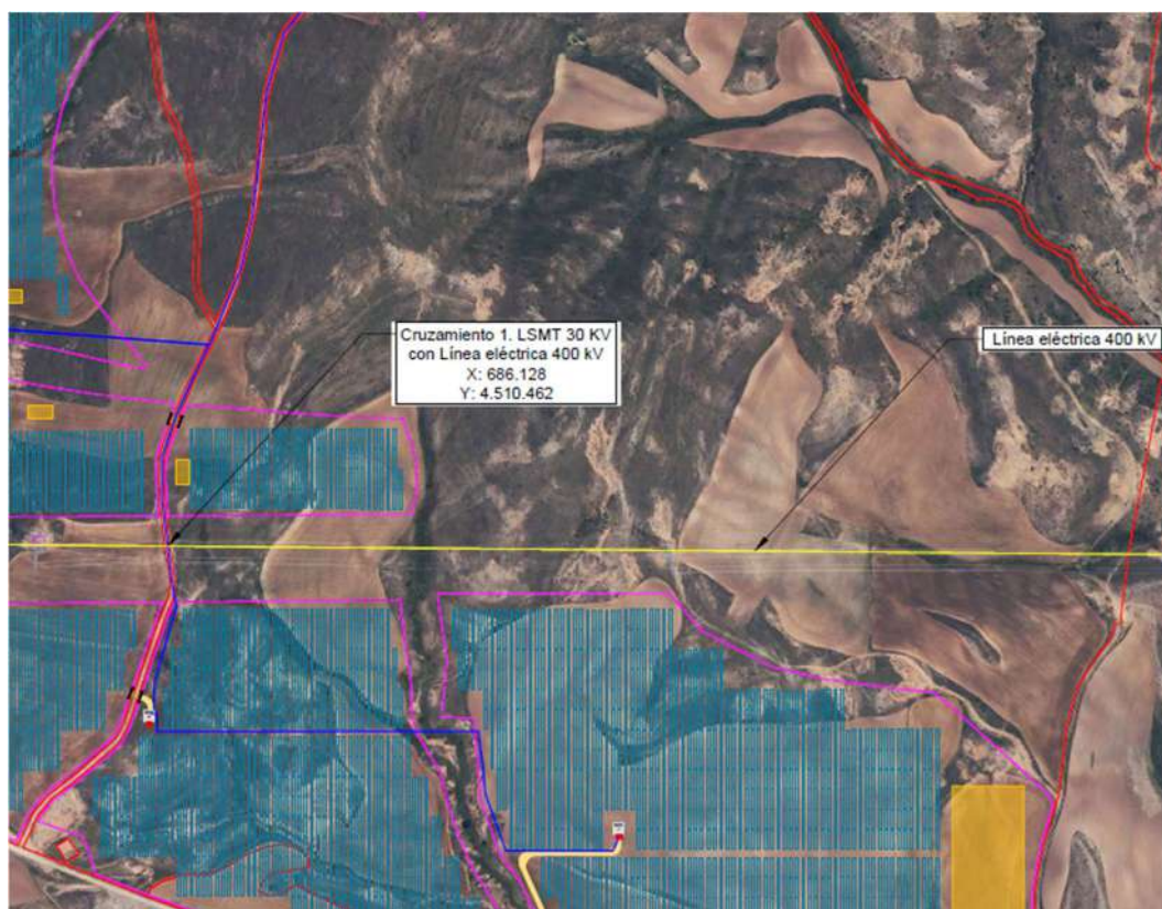
Ilustración 20. Afección líneas eléctricas
