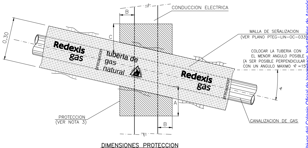
DIMENSIONES PROTECCION
