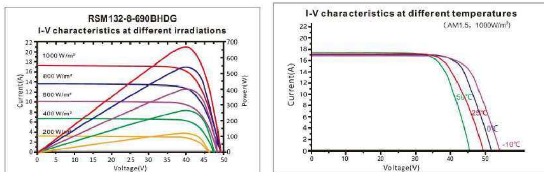
Ilustración 7. Curvas características
