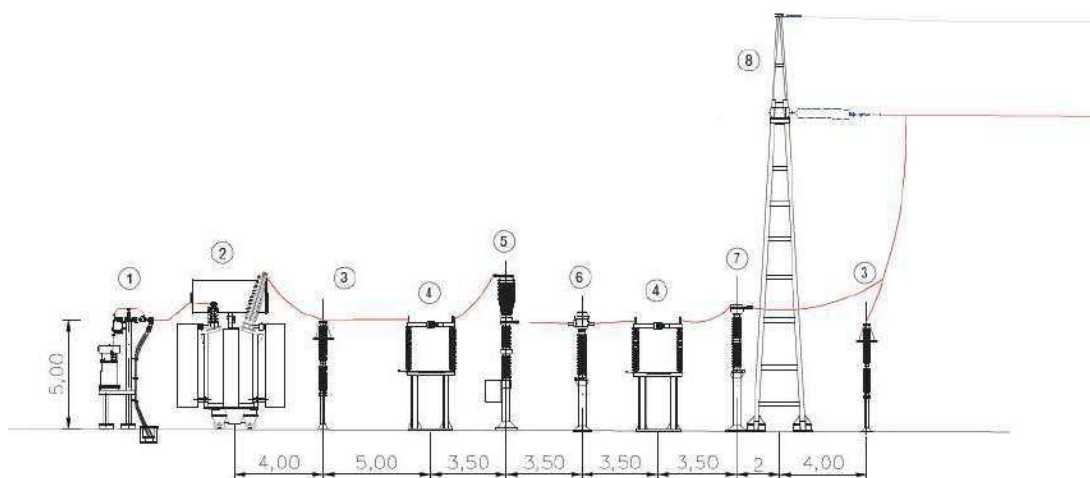
Ilustración 14. Alzado SET
