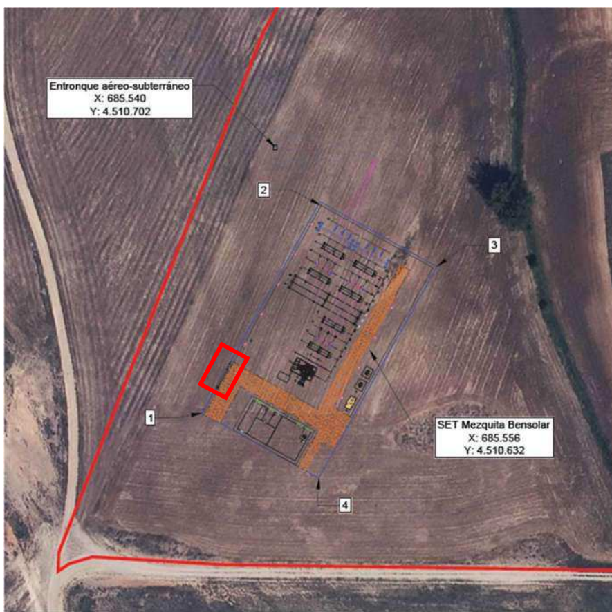
Ilustración 12. Acceso SET
