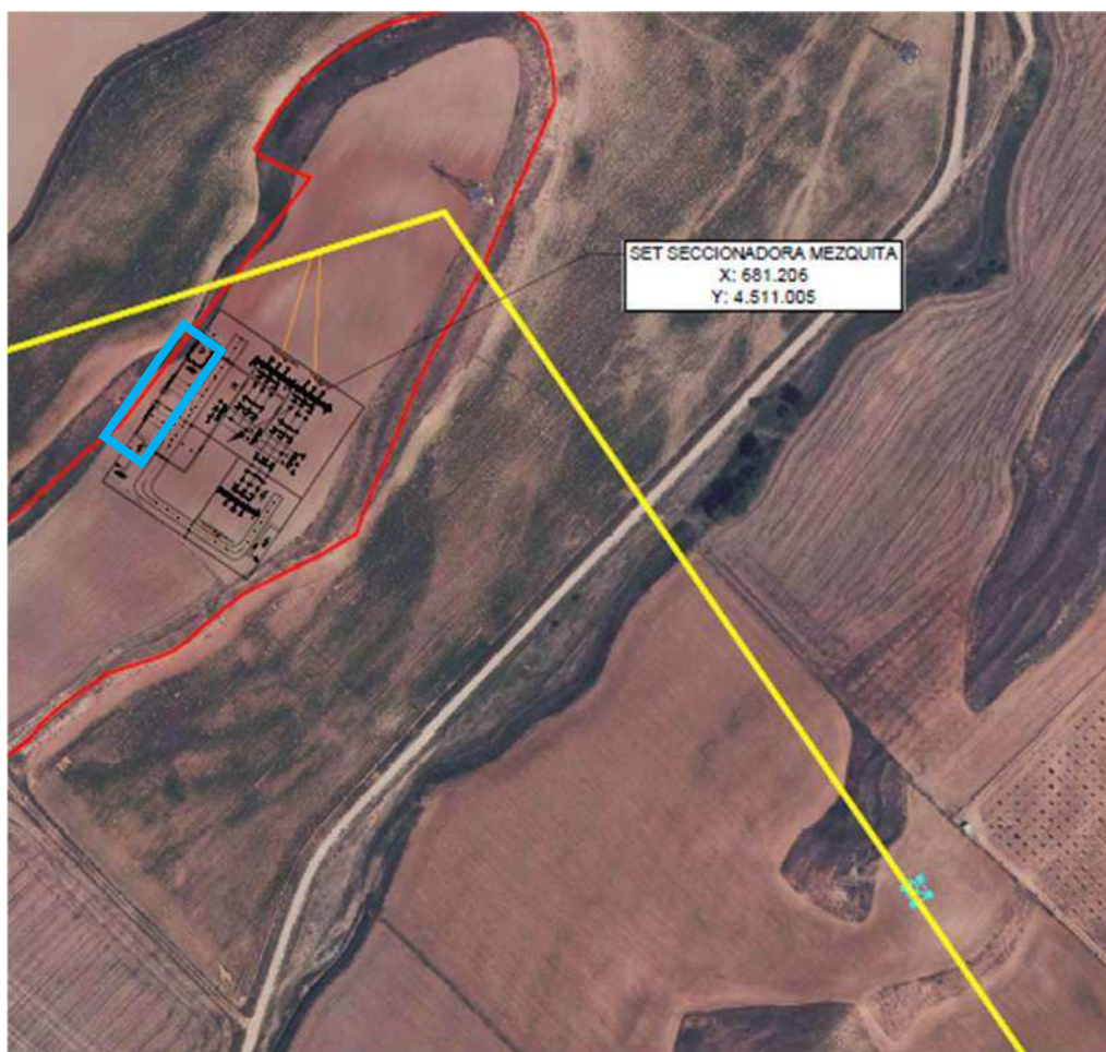
Ilustración 17. Acceso SET
