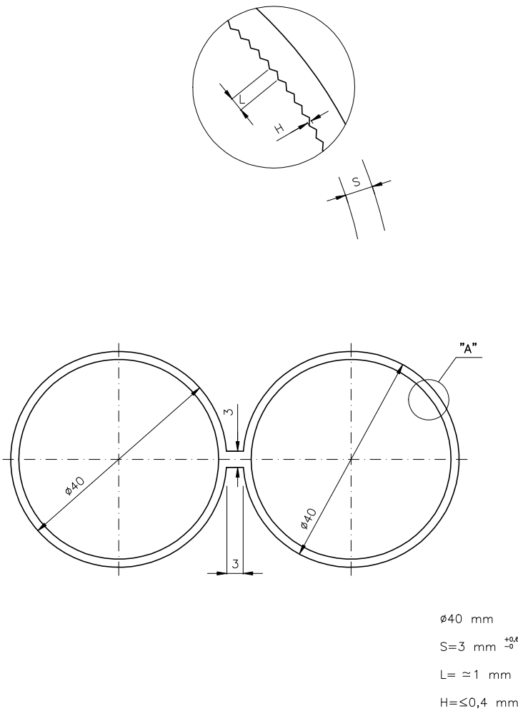
FIGURA Nº 1: SECCION DE BITUBO PEHD \phi 40 \text{ mm}
