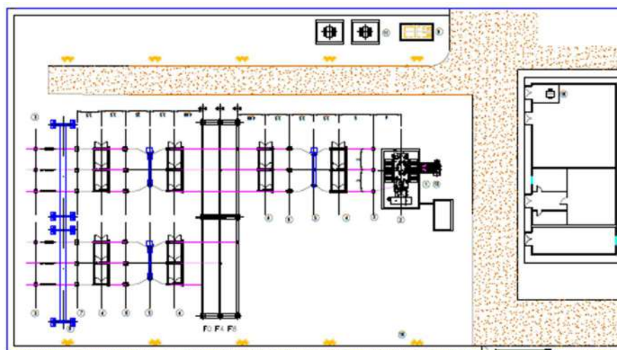
Ilustración 13. Planta SET
