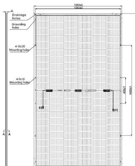
Ilustración 6. Módulo fotovoltaico
