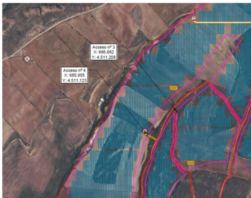
Ilustración 4. Accesos a la planta solar
