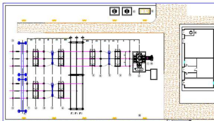
Ilustración 13. Planta SET
