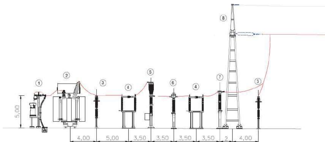
Ilustración 14. Alzado SET
