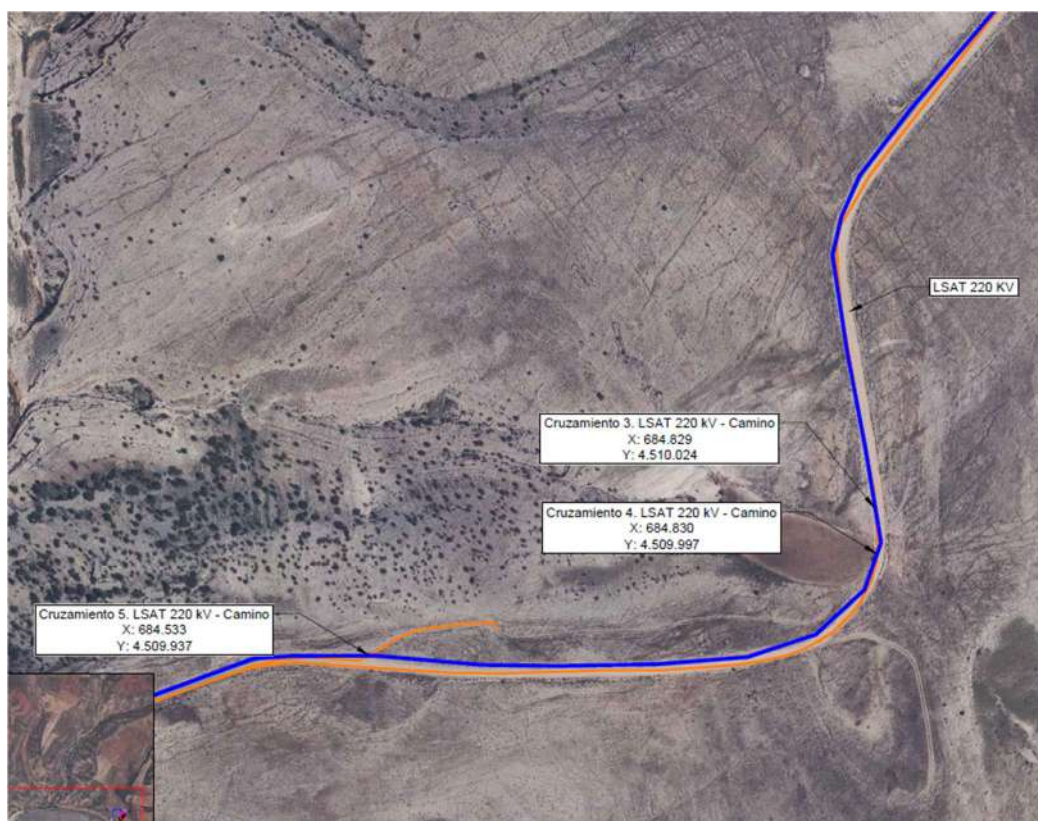
Ilustración 27. Afección a caminos (2/2)
