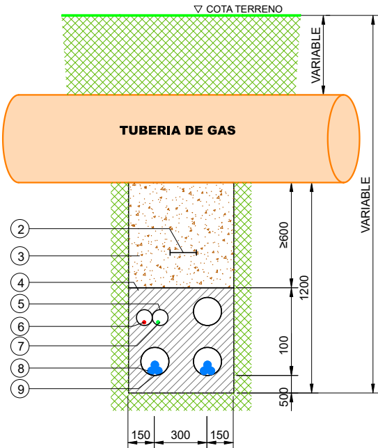
SECCION ZANJA TIPO EN CRUCE DE GASEODUCTO Esc. 1:300
