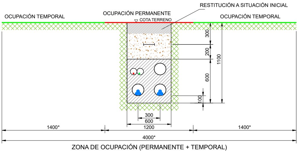
ZANJA DOBLE CIRCUITO Esc. 1:300
