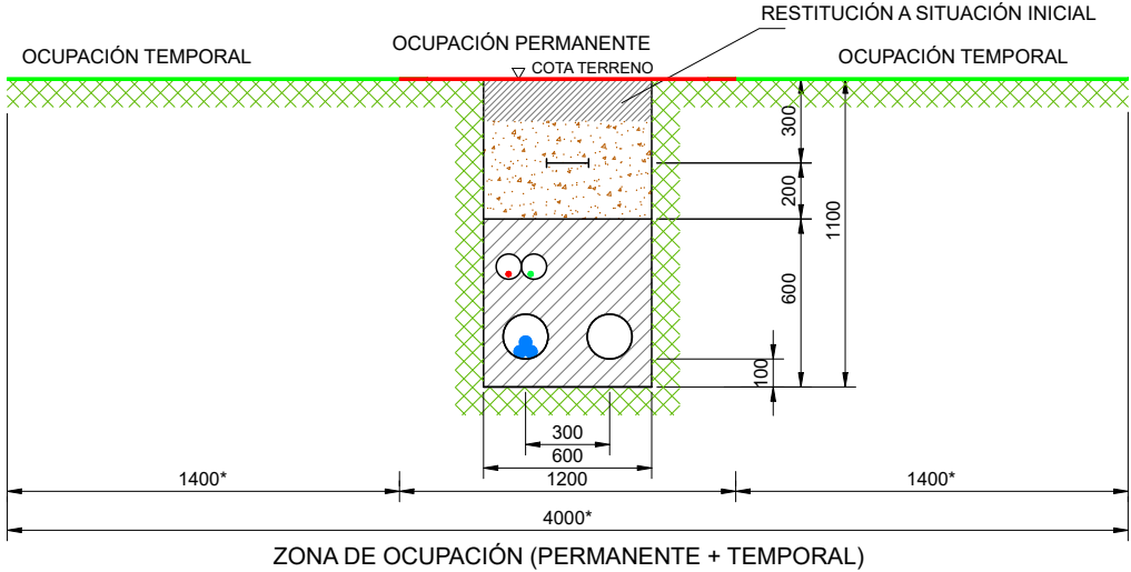
ZANJA SIMPLE CIRCUITO Esc. 1:300
