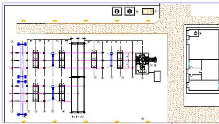
Ilustración 13. Planta SET
