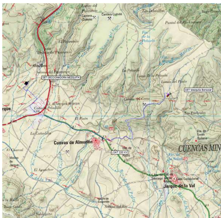
Ilustración 15. Situación LSAT 220 KV
