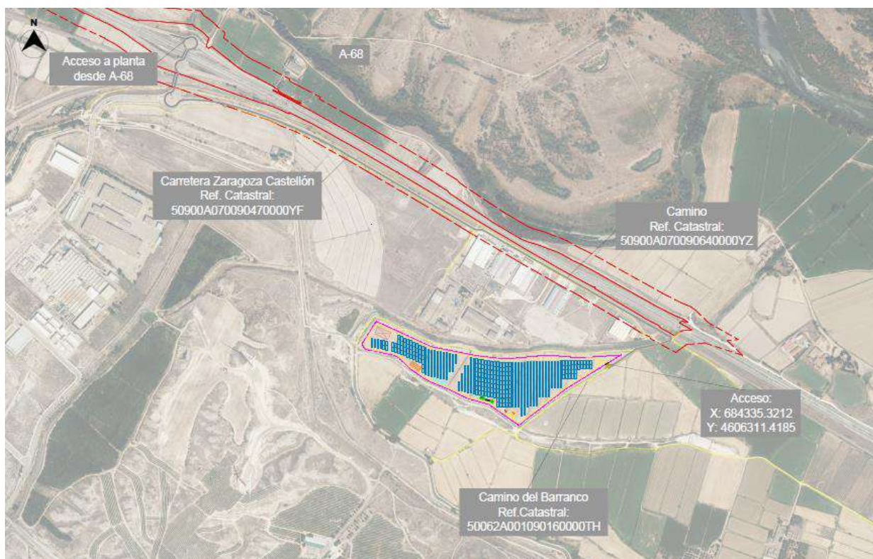
Figura 6: Acceso a la Planta Solar FV
