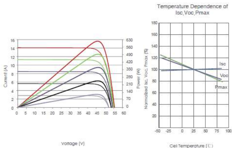
Figura 22: Curvas Características JKM625N-78HL4-BDV
