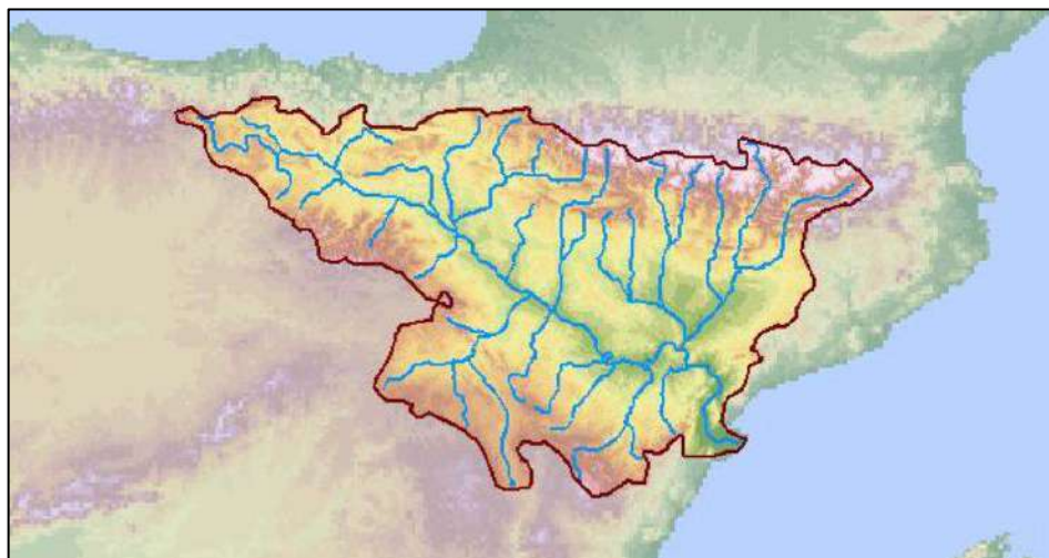
Figura 15: Confederación Hidrográfica del Ebro.
