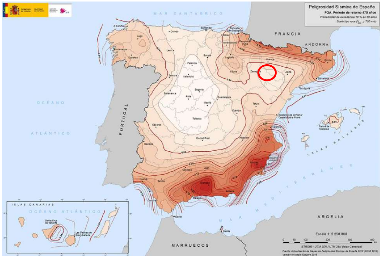
Figura 18: Riesgo Sísmico en la Zona de Actuación
