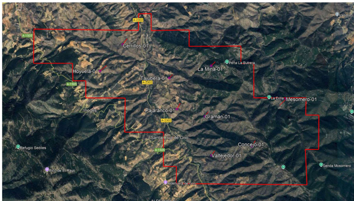
Figura 10. Localización de los sondeos con recuperación de testigo planteados.
