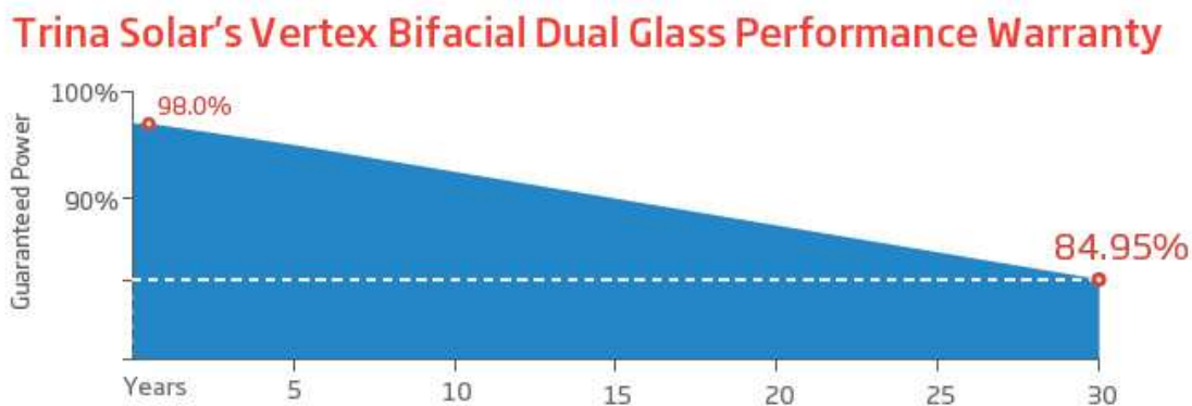
Ilustración 4. Rendimiento y vida útil del módulo fotovoltaico. Fuente: Trina Solar
