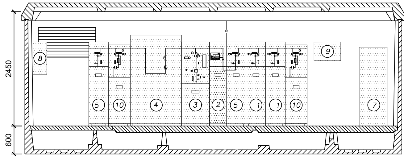
SECCIÓN A-A'
