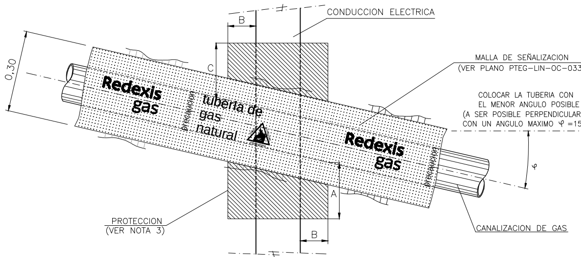
DIMENSIONES PROTECCION
