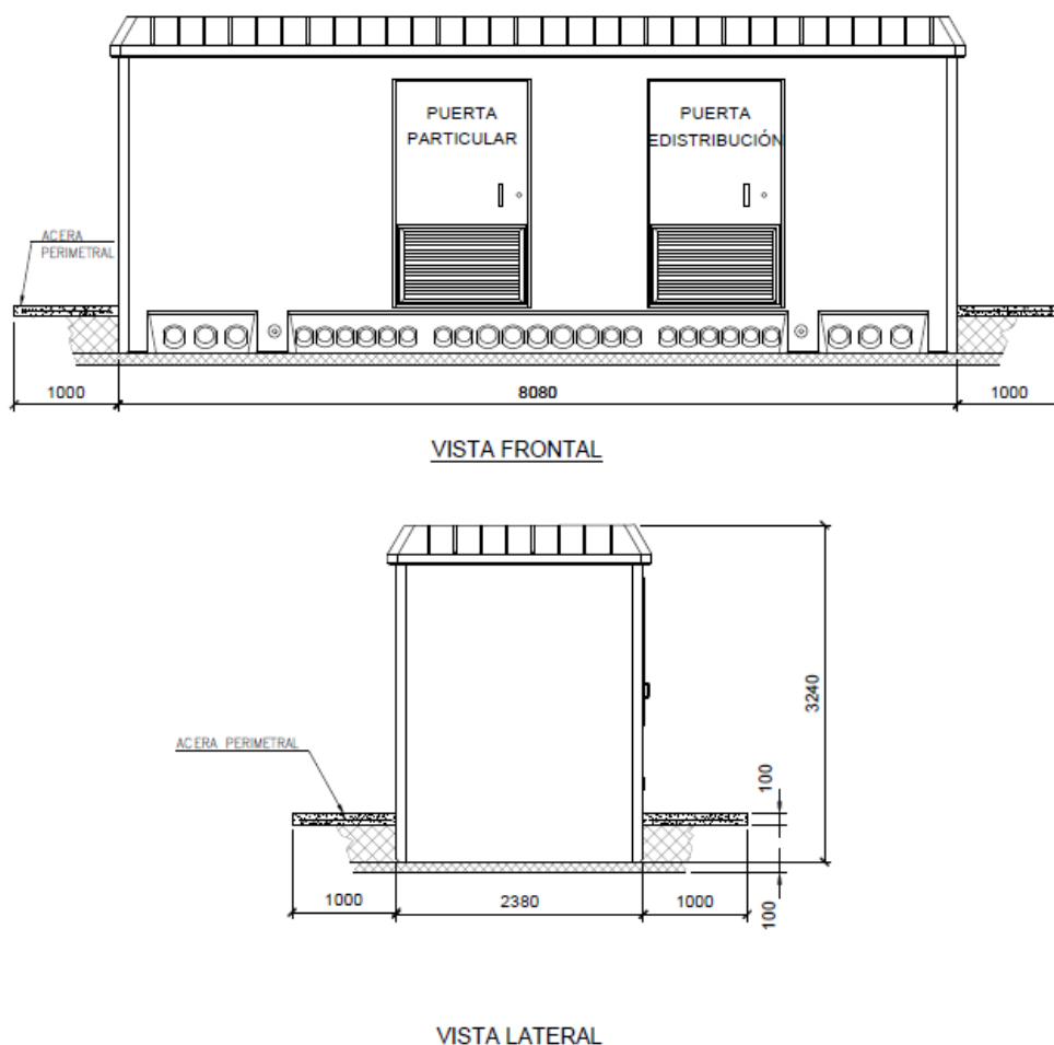
Ilustración. Centro de Seccionamiento 24 kV. Modelo PFU-7. Fuente: Ormazabal
