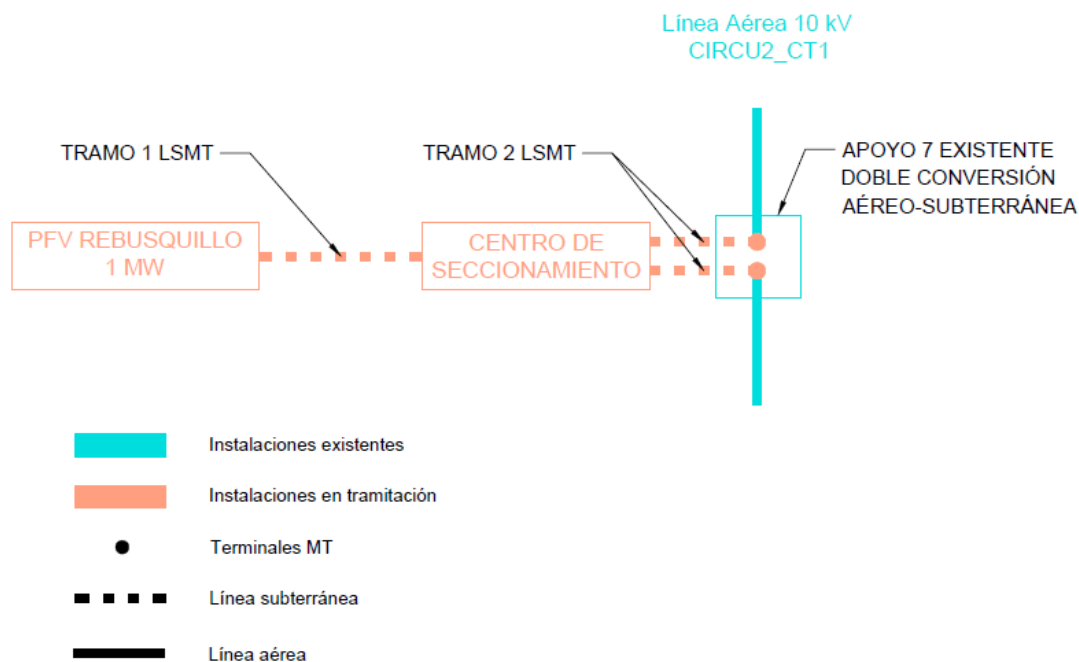
Ilustración 1: Infraestructuras de evacuación del parque fotovoltaico
