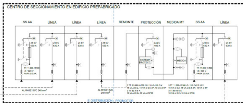
Ilustración. Centro de Seccionamiento. Unifilar
