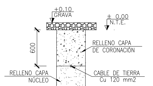
ZANJA CABLE DE TIERRA
