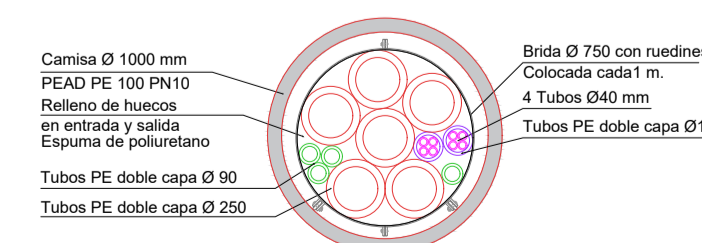
SECCIÓN HINCA L.S.A.T.
