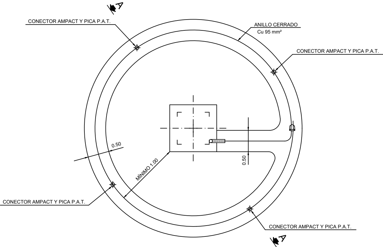
PLANTA APOYO
