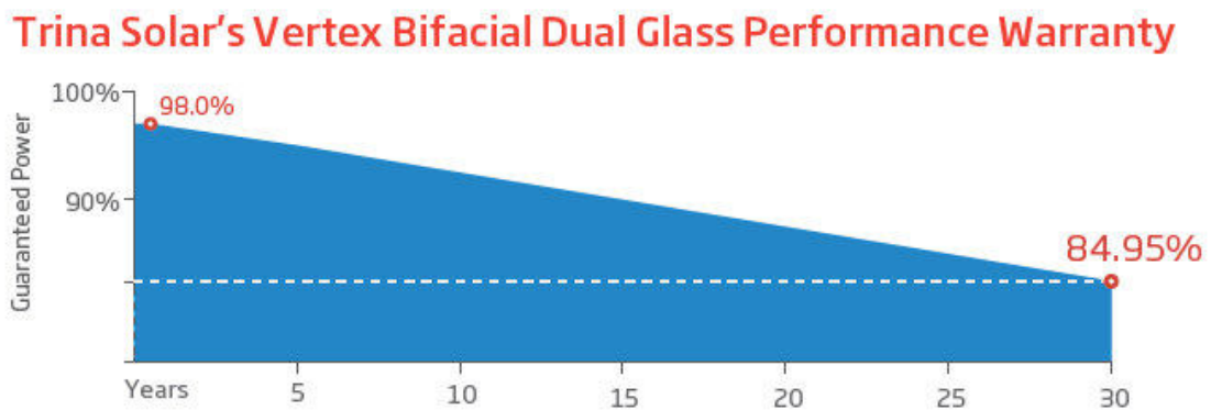
Ilustración 9. Rendimiento y vida útil del módulo fotovoltaico. Fuente: Trina Solar
