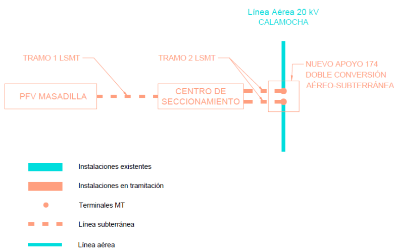
Ilustración 1: Infraestructuras de evacuación del parque fotovoltaico
