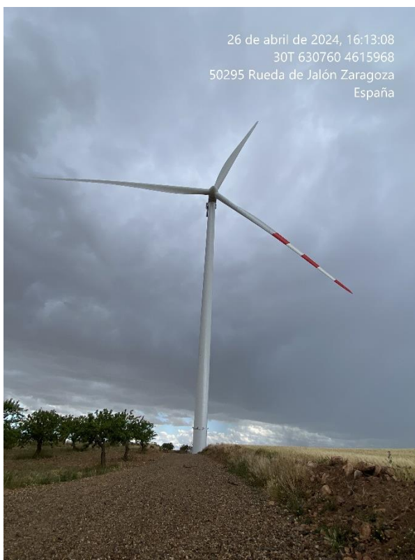
Figura 10: Foto del aerogenerador VAL II - 01 con la medida preventiva de pintado de pala.
