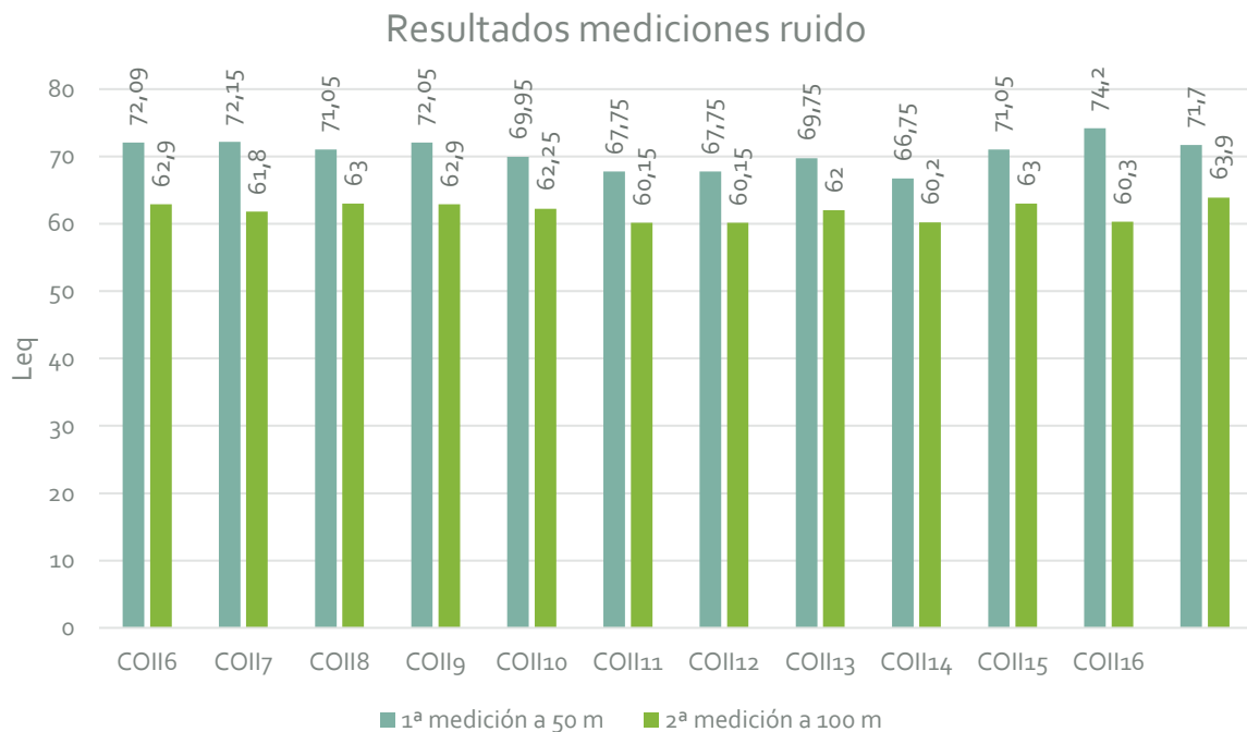
Figura 19. Resultados de las mediciones de ruido en LCII. Fuente: Ideas Medioambientales.
