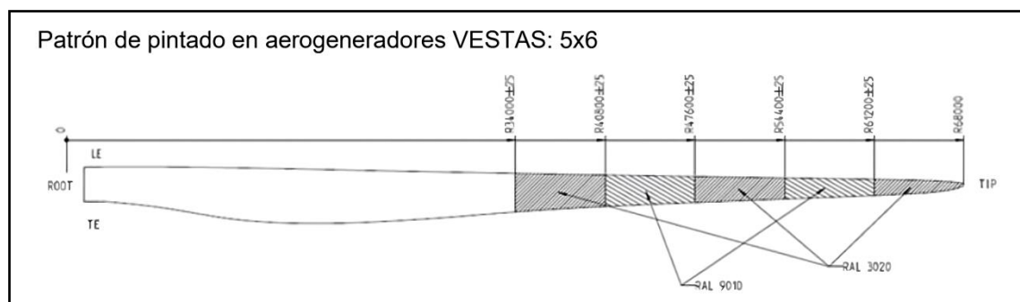
Figura 13: Esquema del patrón de pintado aplicado sobre la pala del aerogenerador en PE “El Tollo”
