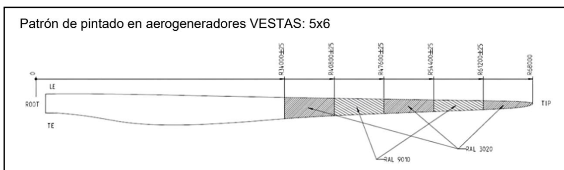
Figura 14: Esquema del patrón de pintado aplicado sobre la pala de los aerogeneradores en PE “El Llano”
