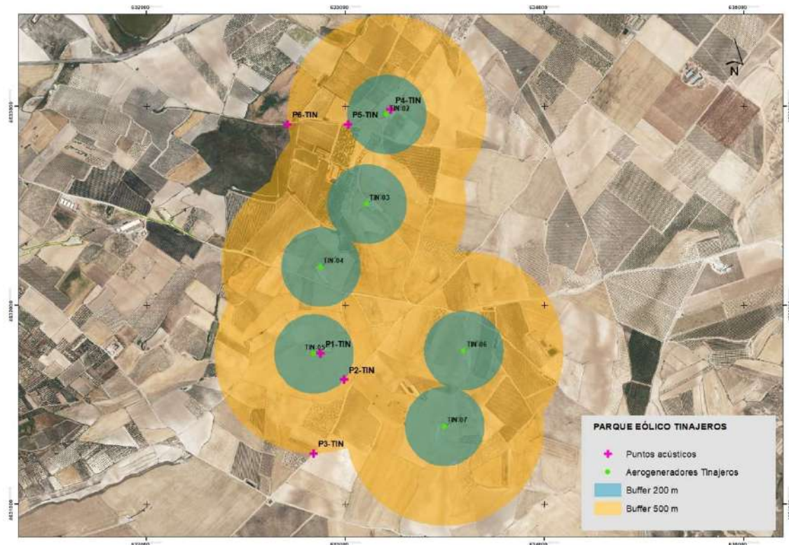
Figura 39: Localización de las estaciones de medición acústica del parque eólico “Tinajeros”.
