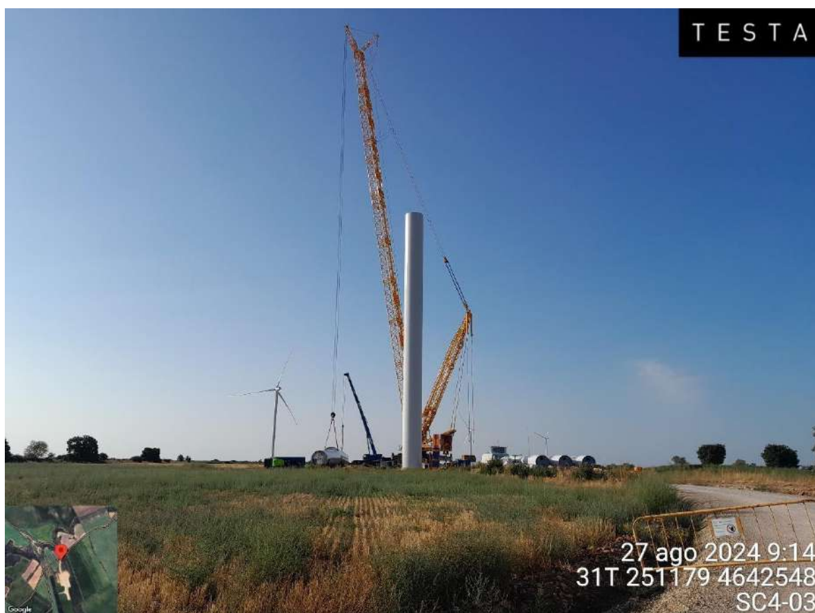
Imagen 2. Montaje de Aerogenerador en la posición SC4-03
