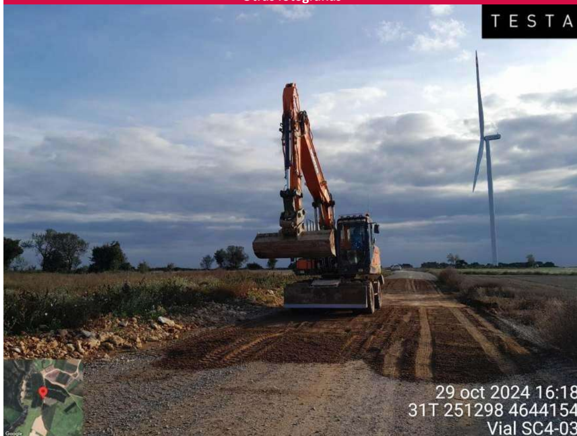
Imagen 1. Trabajos de restauración en el vial de acceso a la posición SC4-03
