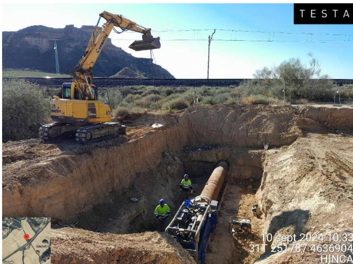
Imagen 2. Perforación en HINCA
