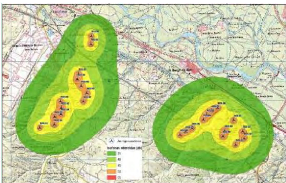
Figura 58. Niveles de presión sonora obtenidos.
