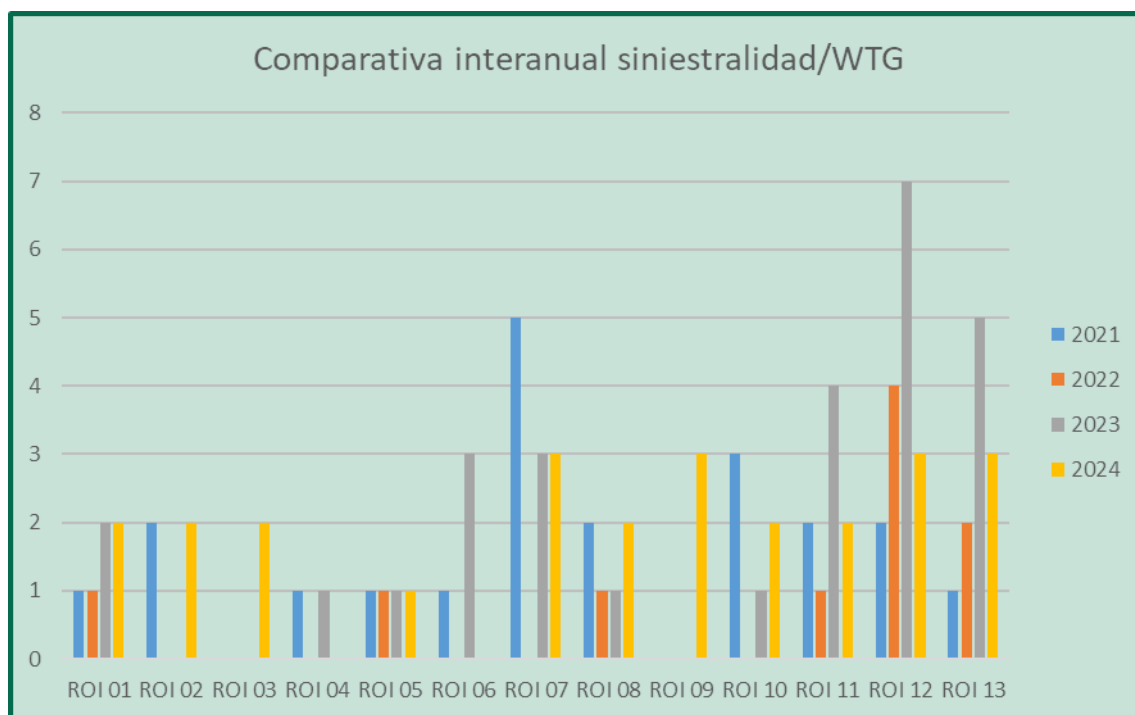
Figura 48. Siniestralidad interanual, durante el 3 er cuatrimestre, por WTG. PE RO I. (2021-2024)
