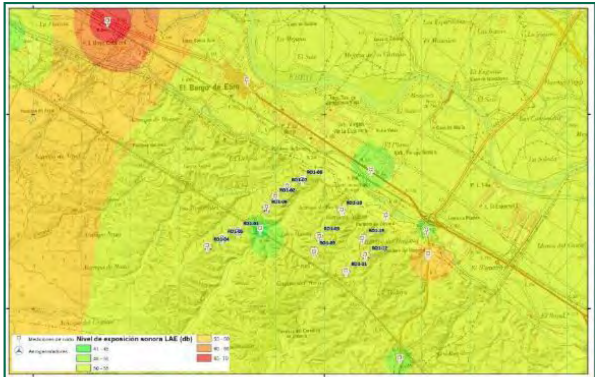
Figura 63. Distribución espacial hallada mediante dos tipos de interpolación diferentes (IDW) de los datos medidos en campo con una velocidad de viento entre 5 y 8 m/s y parques eólicos en funcionamiento.
