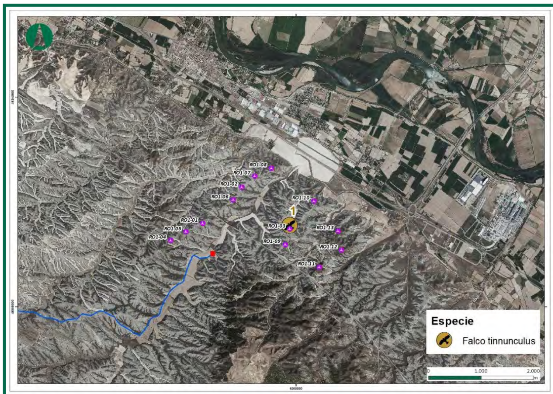
Figura 11. Uso del espacio del cernícalo vulgar ( Falco tinnunculus ), 3º cuatrimestre 2024.
