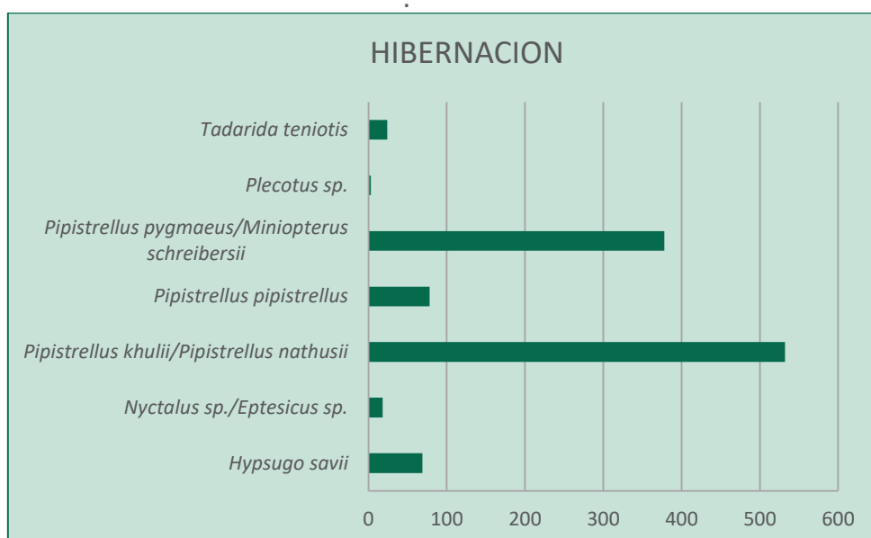
Figura 36. Abundancia de especies/grupo de vocalización durante la etapa de HIBERNACION.
