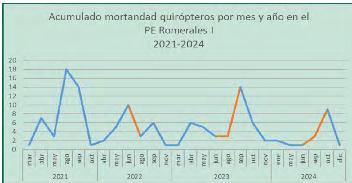
Figura 57. Mortandad quirópteros agosto-noviembre 2022-2024. (Línea roja corresponde con el periodo de parada para quirópteros).
