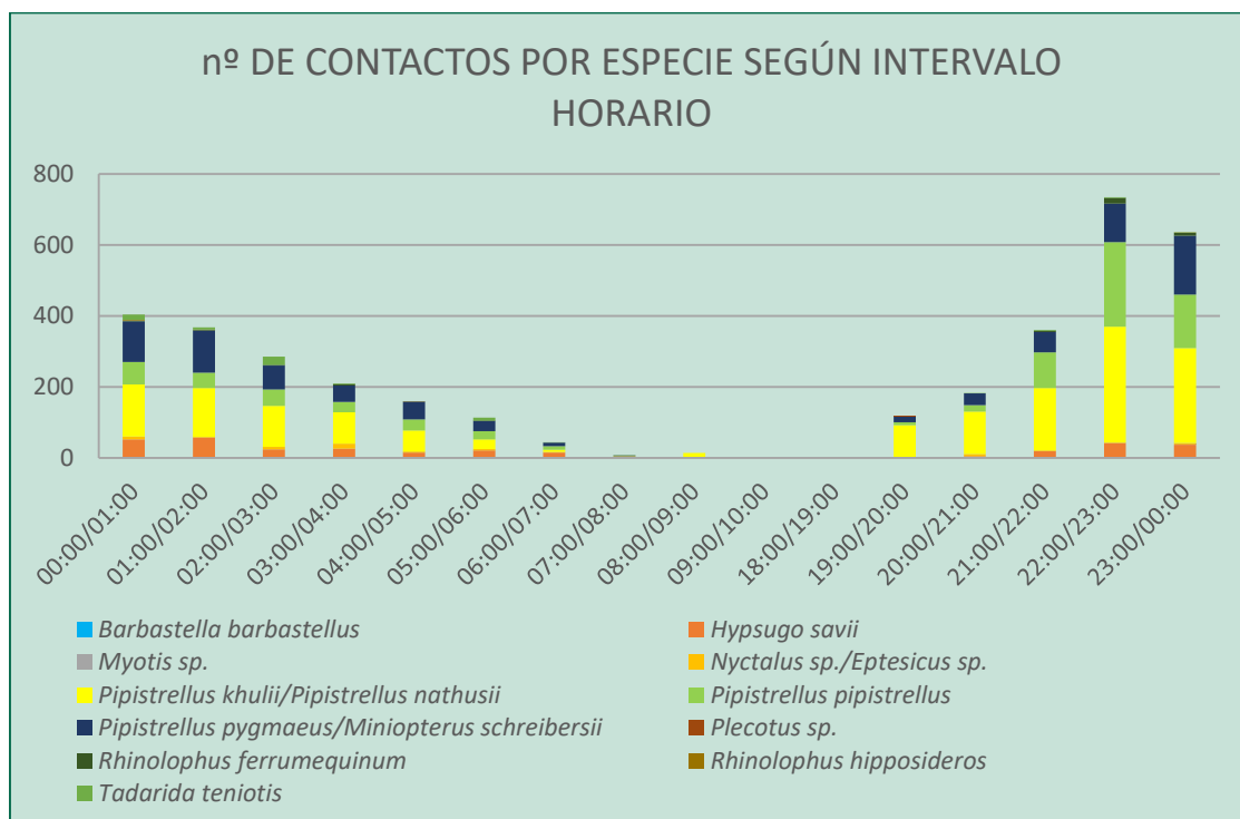
Figura 30. Registros totales de contactos, por especies y por intervalos. Periodo anual 2024.
