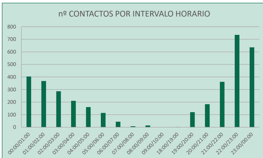
Figura 28. Registros totales en función de la hora. 2024.
