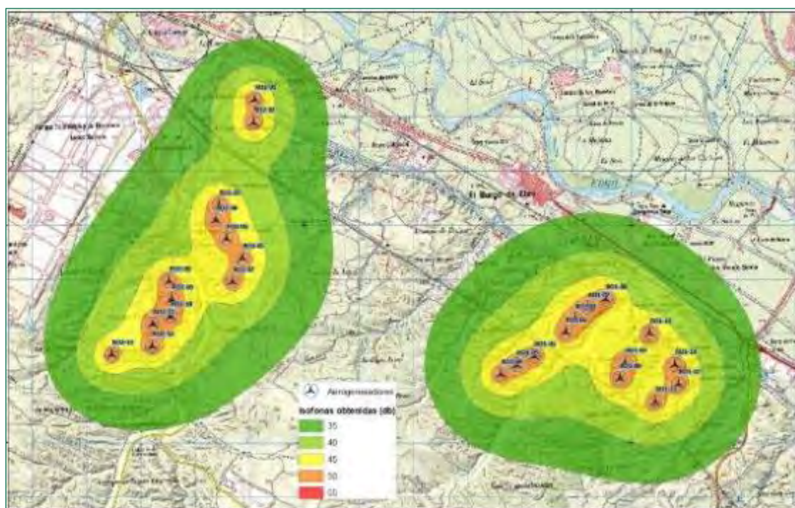
Figura 56. Niveles de presión sonora obtenidos.
