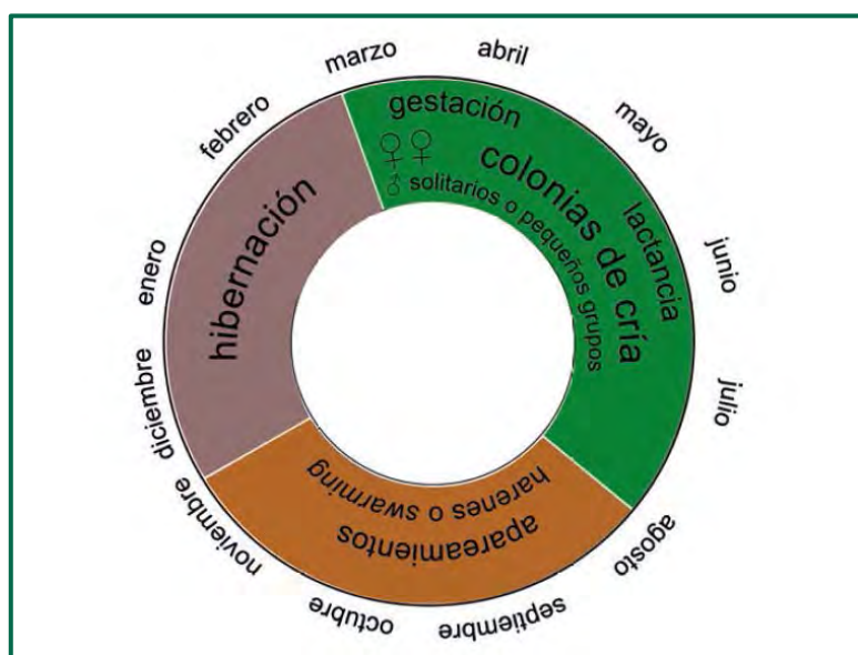
Figura 29. Ciclo biológico anual típico de los murciélagos de zonas templadas. Las fechas que delimitan los diferentes periodos varían dependiendo de la climatología de cada región.
