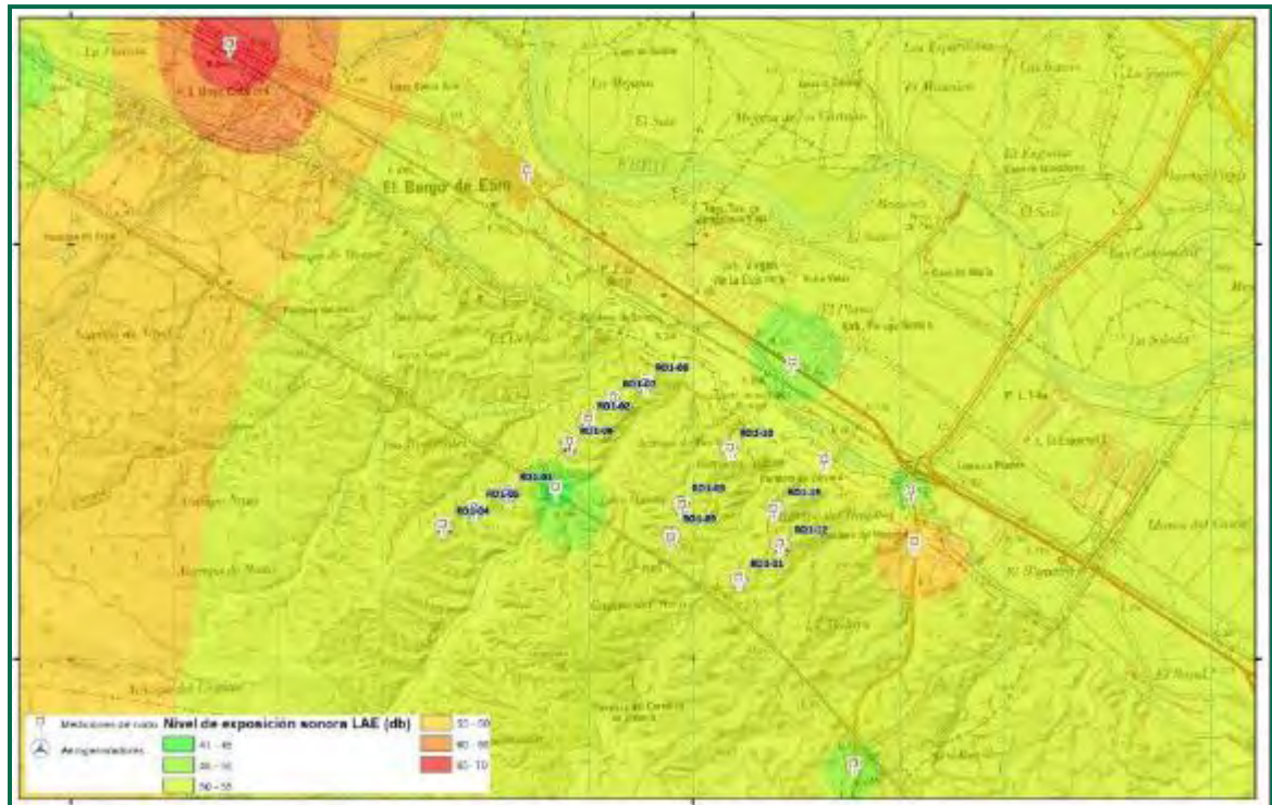
Figura 61. Distribución espacial hallada mediante dos tipos de interpolación diferentes (IDW) de los datos medidos en campo con una velocidad de viento entre 5 y 8 m/s y parques eólicos en funcionamiento.
