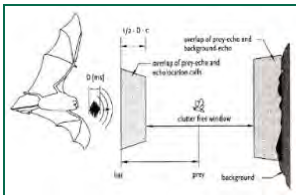
Figura 20. Delante de cada murciélago que esté utilizando la ecolocalización se extiende una "ventana ciega", puesto que el eco que retorna lo hace mientras el murciélago aún está emitiendo los pulsos de llamada. Una zona similar, en la que el murciélago puede apenas detectar ecos débiles, se asocia con cualquier superficie reflectante. Tan sólo entre ellos existe una "ventana sin interferencias" (clutter-free window), en la cual el murciélago puede detectar los ecos débiles de pequeños insectos.
