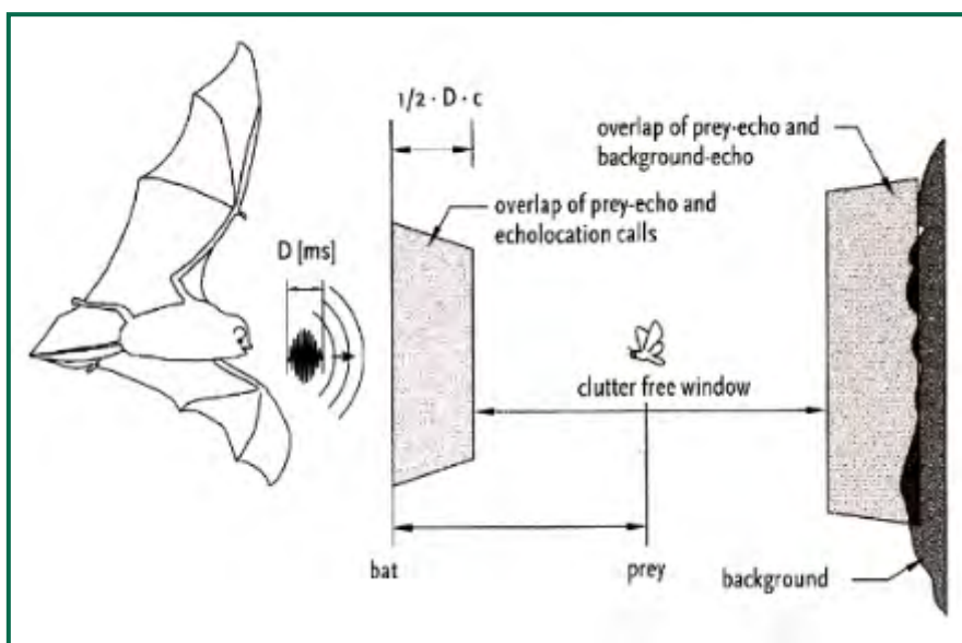
Figura 14. Delante de cada murciélago que esté utilizando la ecolocalización se extiende una "ventana ciega", puesto que el eco que retorna lo hace mientras el murciélago aún está emitiendo los pulsos de llamada. Una zona similar, en la que el murciélago puede apenas detectar ecos débiles, se asocia con cualquier superficie reflectante. Tan sólo entre ellos existe una "ventana sin interferencias" (clutter-free
