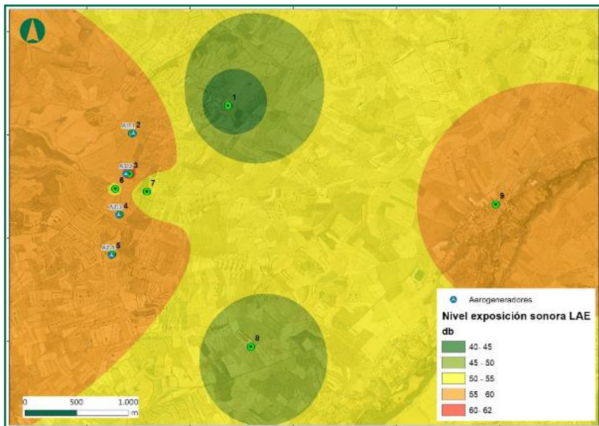
Figura 23. Puntos de medición y distribución espacial hallada mediante dos tipos de interpolación diferentes (IDW) de los datos medidos en campo con una velocidad de viento entre 5 y 8 m/s y parques eólicos en funcionamiento.
