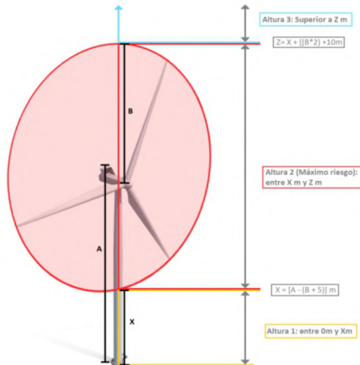
Figura 10: Esquema que muestra el rango de alturas de vuelo definidas en función de su riesgo respecto a los aerogeneradores.
