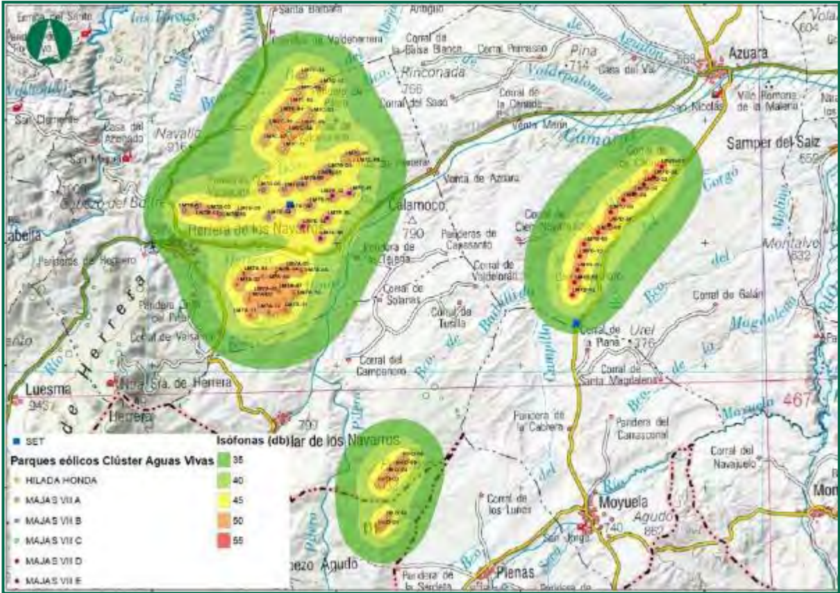
Figura 67. Niveles de presión sonora obtenidos.
