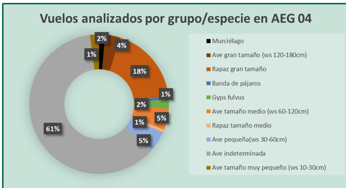
Figura 59. Porcentaje de vuelos por especie/grupo AG04.
