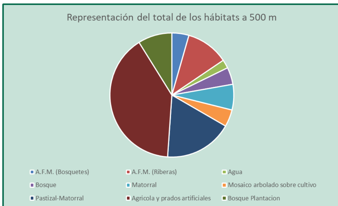
Figura 36. Porcentaje de los hábitats que abarca las estaciones a 500 m.
