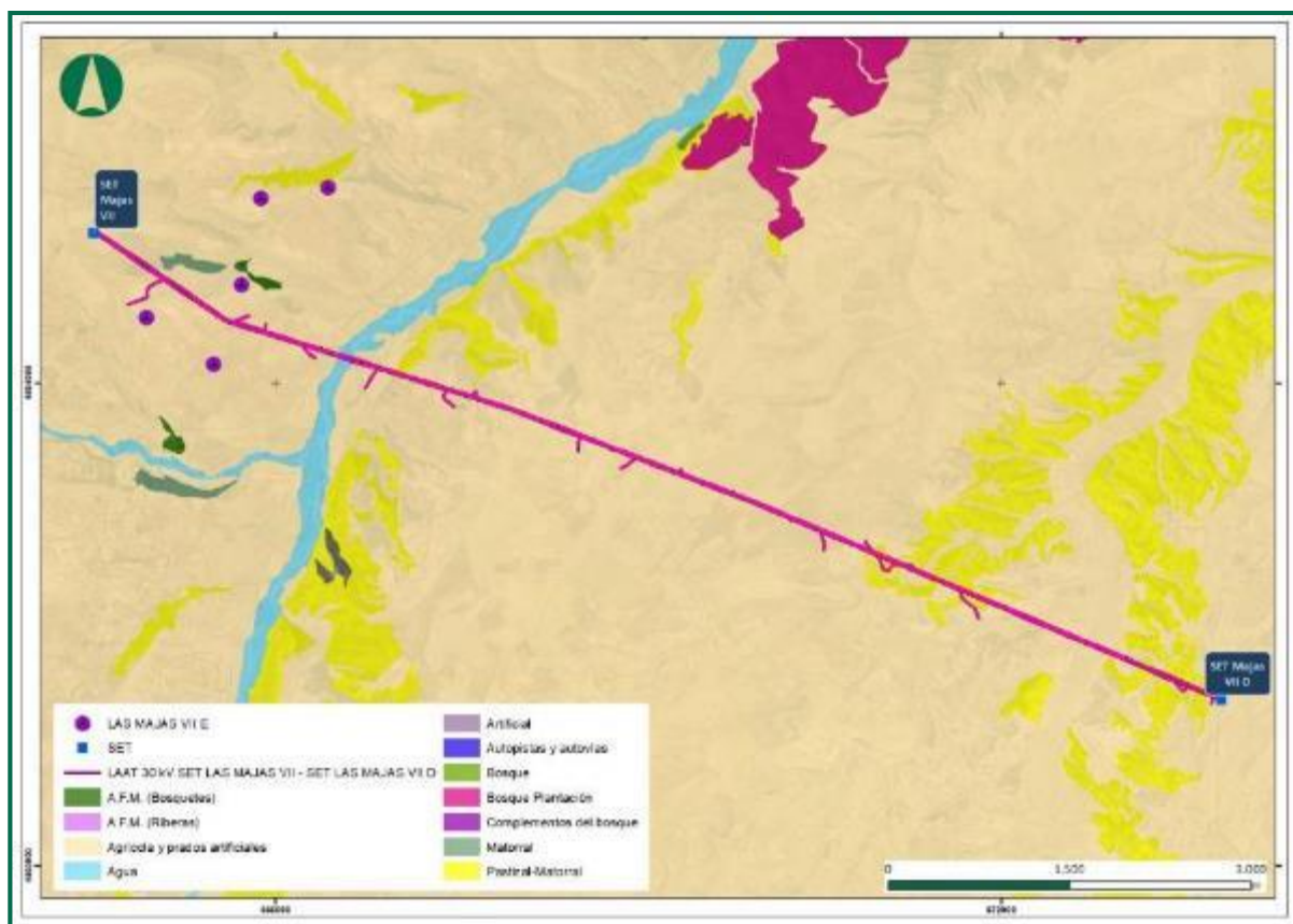
Figura 49. Mapa Forestal de España. Escala 1:50.000.
