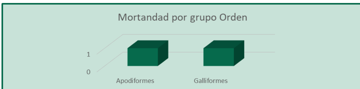
Figura 50. Mortalidad registrada por especie para el periodo en estudio.
