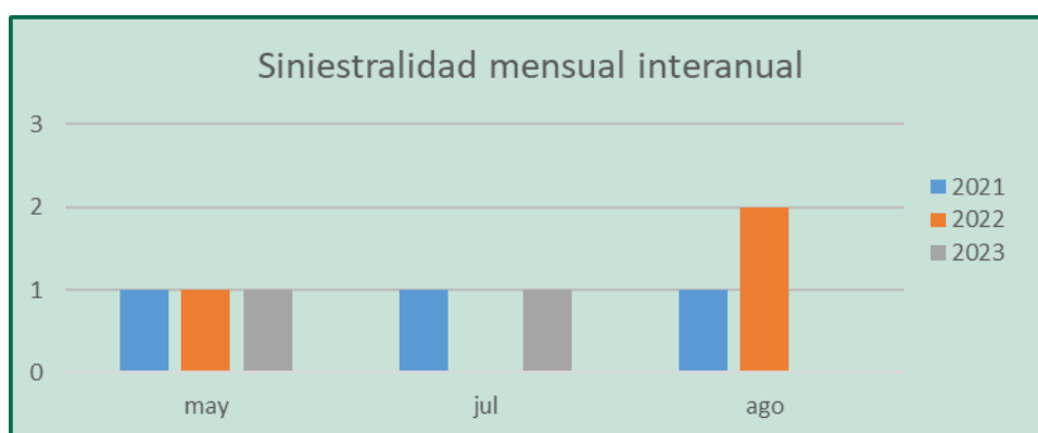
Figura 46. Mortalidad interanual para el 2º cuatrimestre por mes, en el PE Las Majas VII E.
