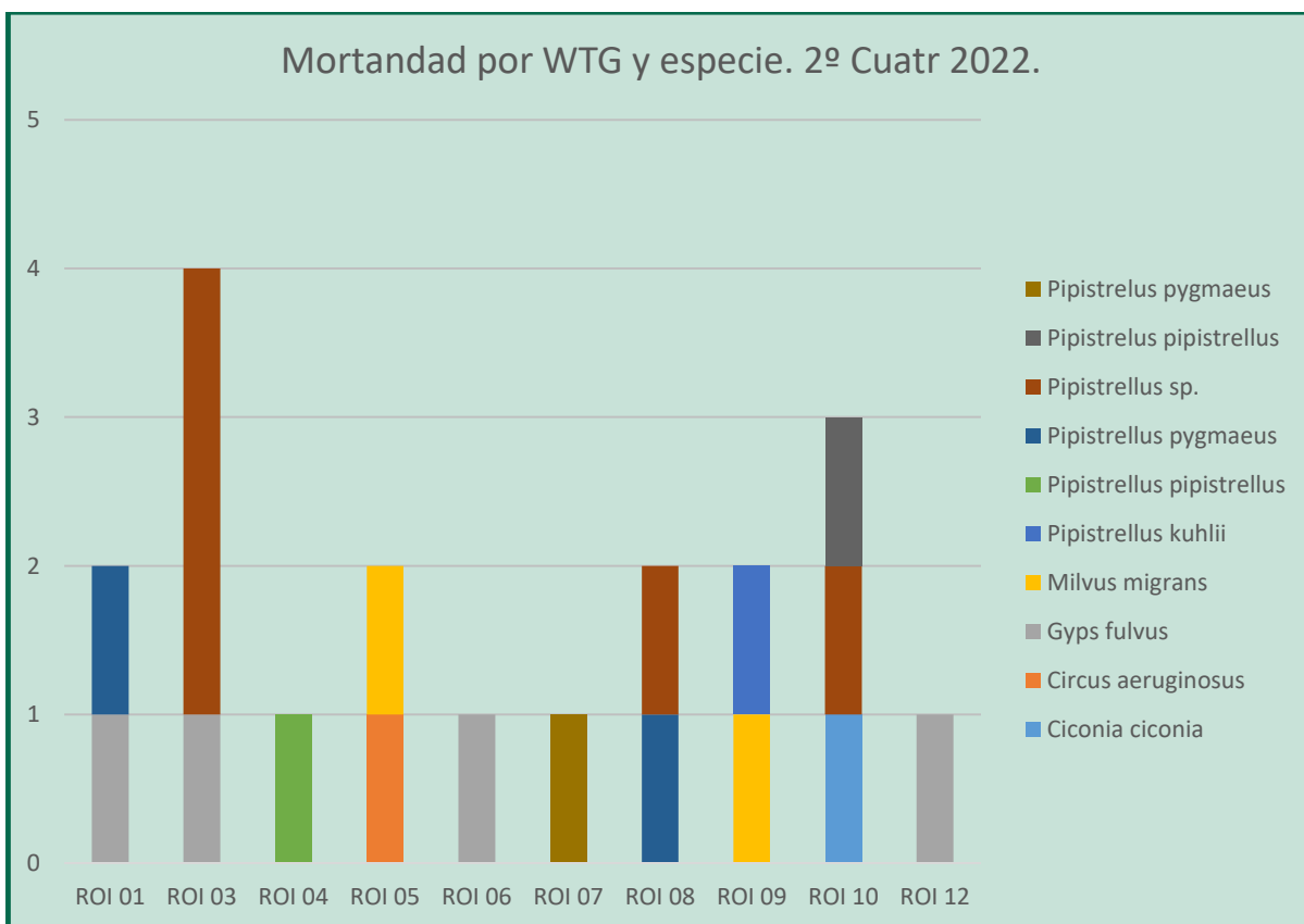
Figura 43. Mortalidad por especie registrada en cada aerogenerador del 2º cuatr. 2022 en el PE Las Majas VII E.
