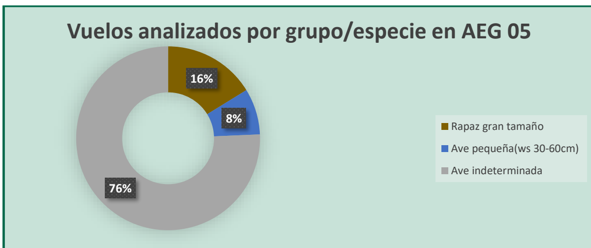
Figura 60. Porcentaje de vuelos por especie/grupo AG05.
