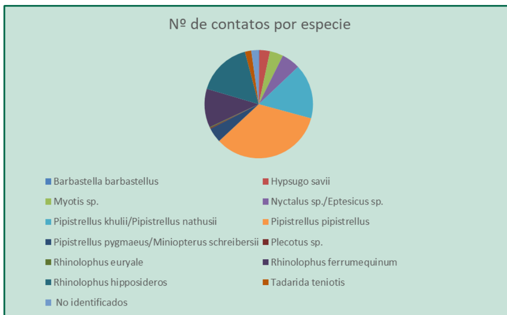
Figura 31. Registros totales de las diferentes especies identificadas.
