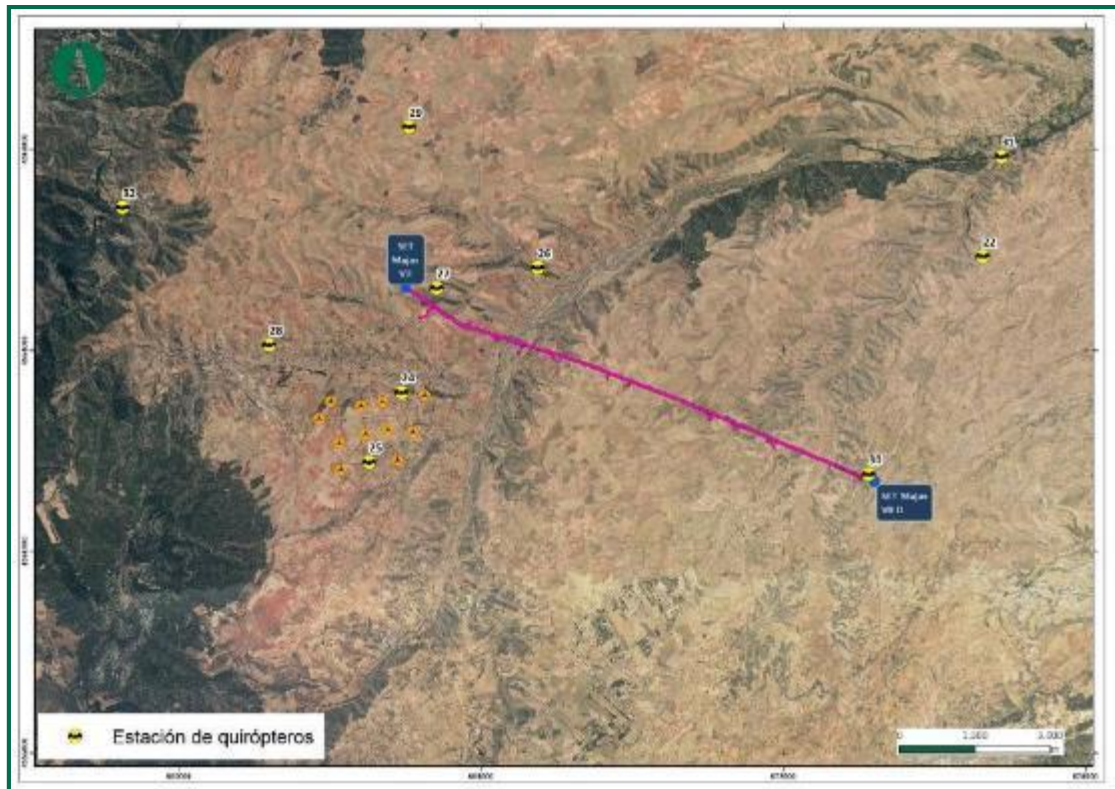
Figura 32. Estaciones de grabación de quiroptero.
