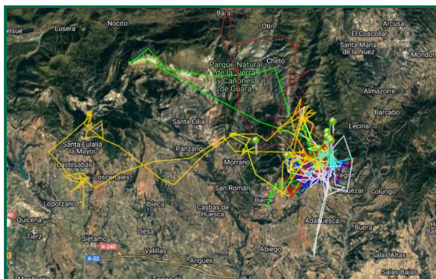
Figura 57. Dispersión de los ejemplares liberados en 2023 durante los primeros días y de “Alquezar”, macho liberado en 2022.
