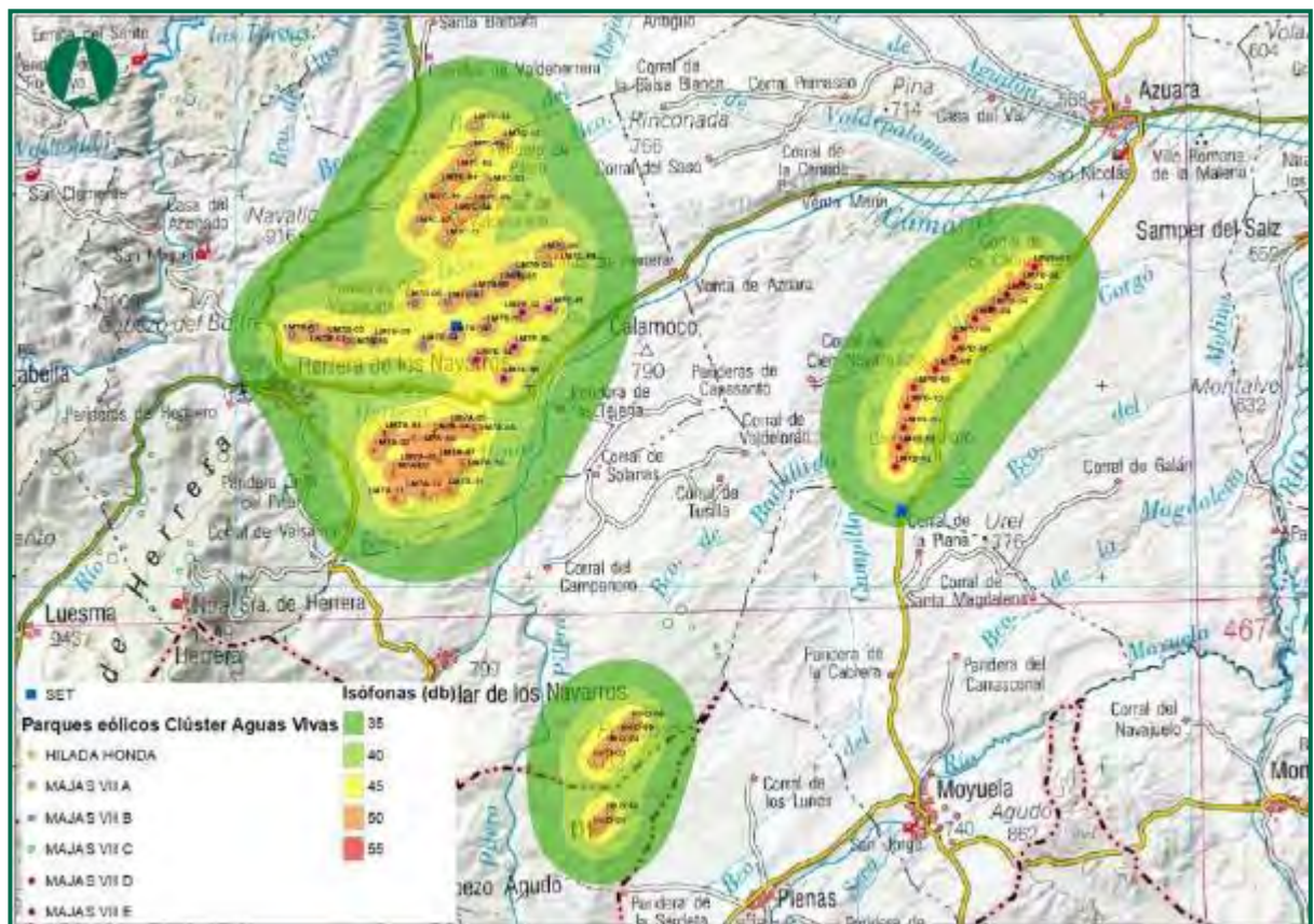
Figura 56. Niveles de presión sonora obtenidos.
