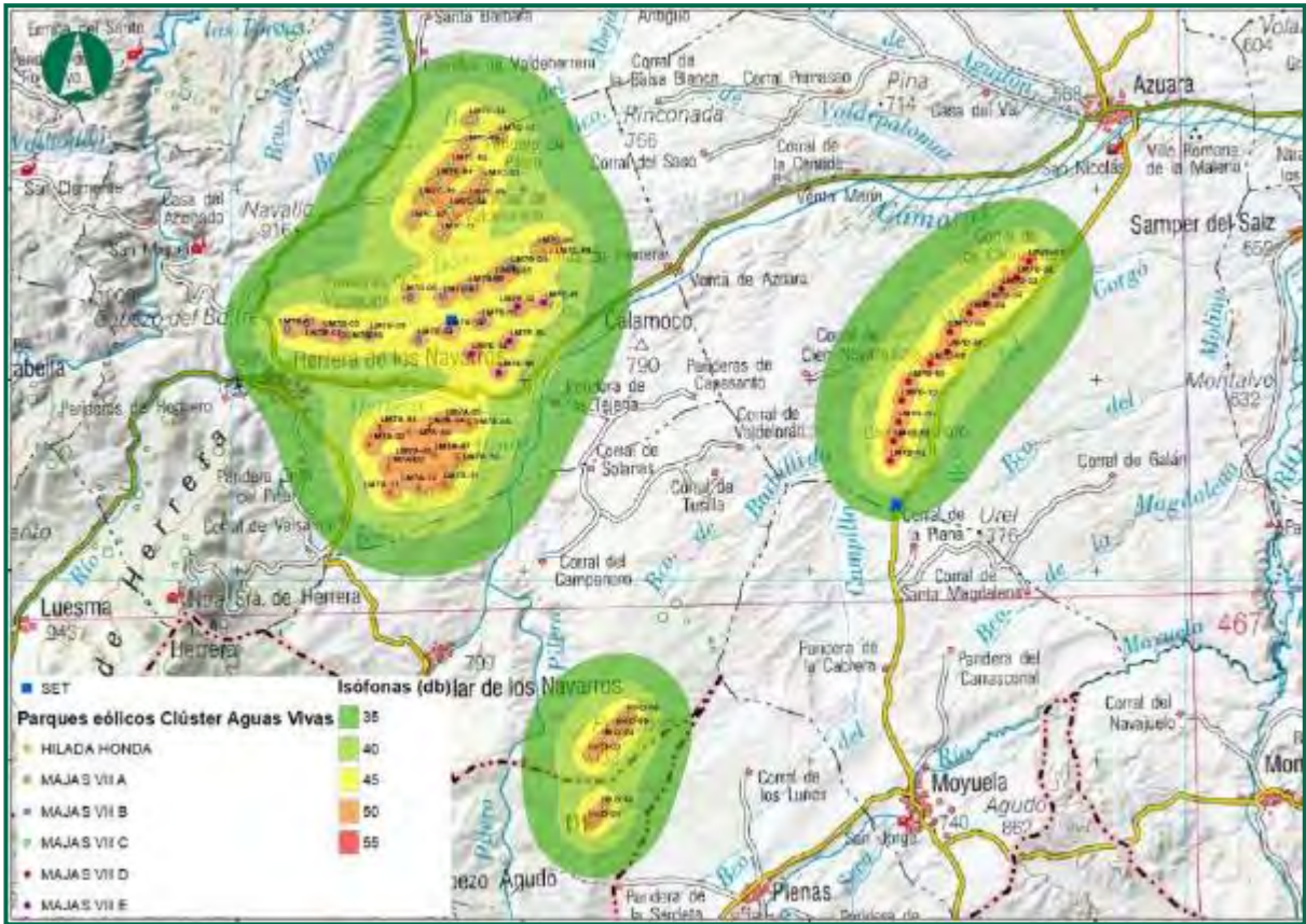
Figura 58. Niveles de presión sonora obtenidos.
