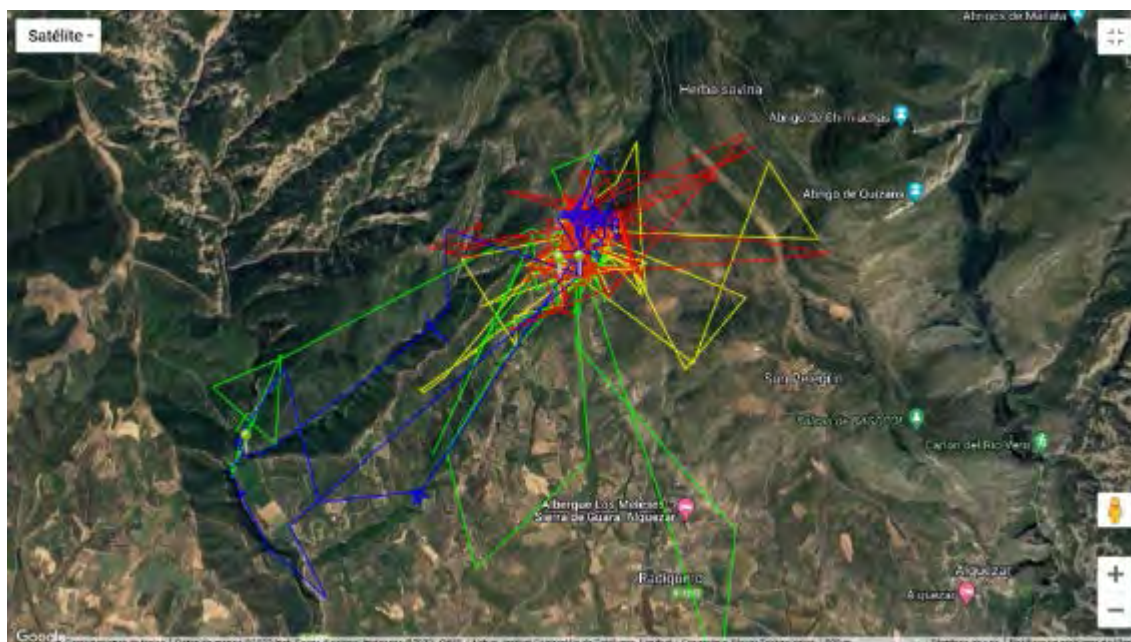
Figura 61. Dispersión de los ejemplares liberados en 2022 durante los primeros días.
