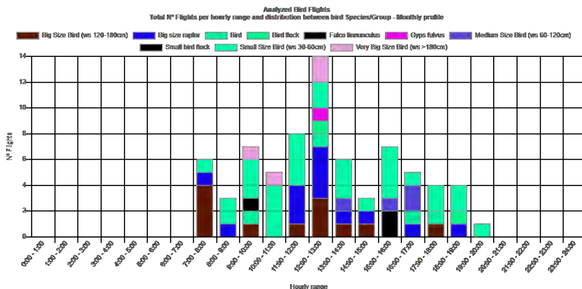
Figura 55. Vuelos analizados por especie, perfil cuatrimestral por horas. WTG LM7C-13 Fuente: DtBird.
