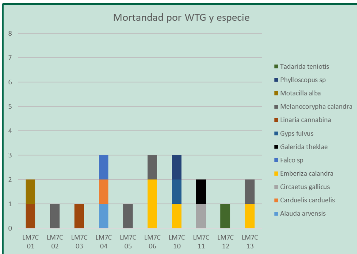
Figura 44. Mortalidad por especie registrada en cada aerogenerador para el periodo en estudio en el PE Las Majas VII C (2024).
