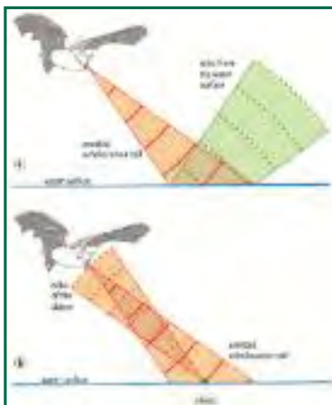
Figura 32. Cazar sobre una superficie suave (como la superficie del agua) conlleva la ventaja de que el impacto del sonido sobre la superficie se refleja en una dirección alejada del murciélago (a) y sólo recibe el eco de vuelta si un objeto, p.ej. una presa, es interceptada (b).
