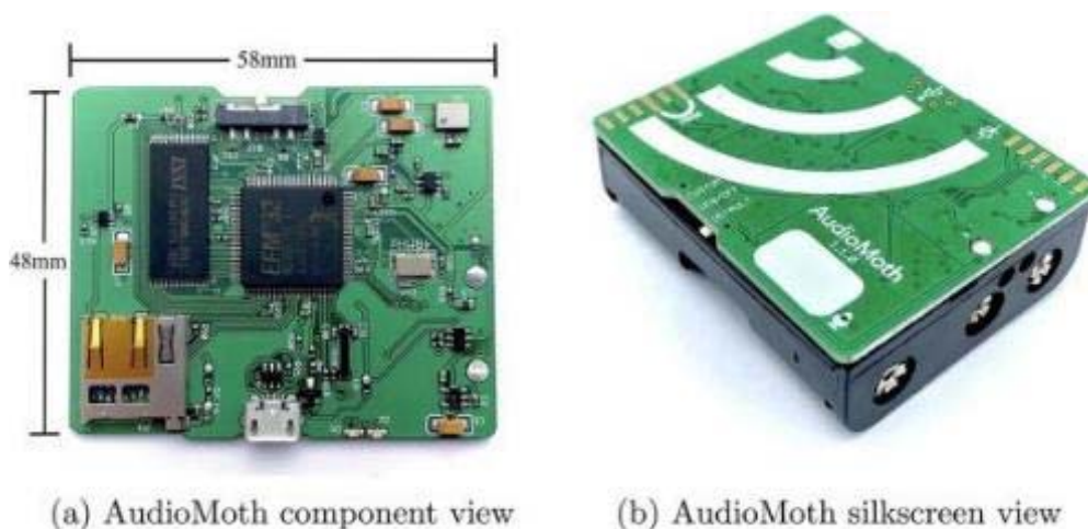
Figura 26. Audiomoth: vista del interior (a) y del exterior (b). Fuente: Hill et al. (2019).
