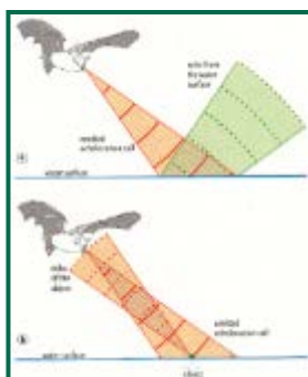
Figura 30. Cazar sobre una superficie suave (como la superficie del agua) conlleva la ventaja de que el impacto del sonido sobre la superficie se refleja en una dirección alejada del murciélago (a) y sólo recibe el eco de vuelta si un objeto, p.ej. una presa, es interceptada (b).
