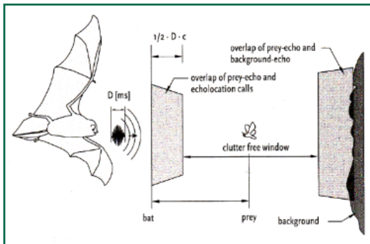
Figura 29. Delante de cada murciélago que esté utilizando la ecolocalización se extiende una "ventana ciega", puesto que el eco que retorna lo hace mientras el murciélago aún está emitiendo los pulsos de llamada. Una zona similar, en la que el murciélago puede apenas detectar ecos débiles, se asocia con cualquier superficie reflectante. Tan sólo entre ellos existe una "ventana sin interferencias" (clutter-free window), en la cual el murciélago puede
