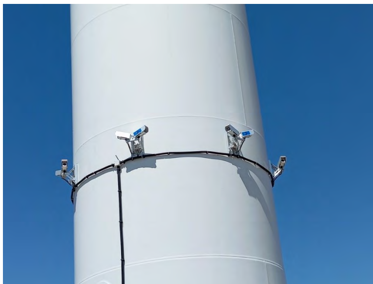
Fotografías 17. Cámaras en los aerogeneradores
