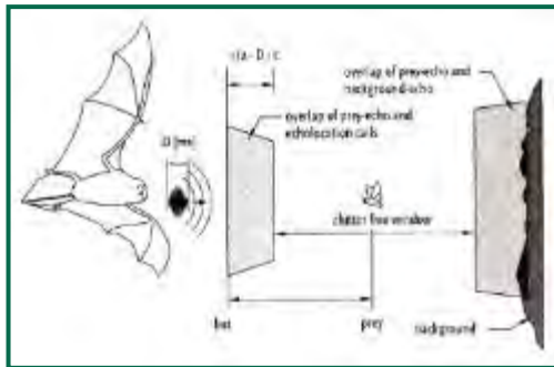
Figura 16. Delante de cada murciélago que esté utilizando la ecolocalización se extiende una "ventana ciega", puesto que el eco que retorna lo hace mientras el murciélago aún está emitiendo los pulsos de llamada. Una zona similar, en la que el murciélago puede apenas detectar ecos débiles, se asocia con cualquier superficie reflectante. Tan sólo entre ellos existe una "ventana sin interferencias" (clutter-free window), en la cual el murciélago puede detectar los ecos débiles de pequeños insectos.
