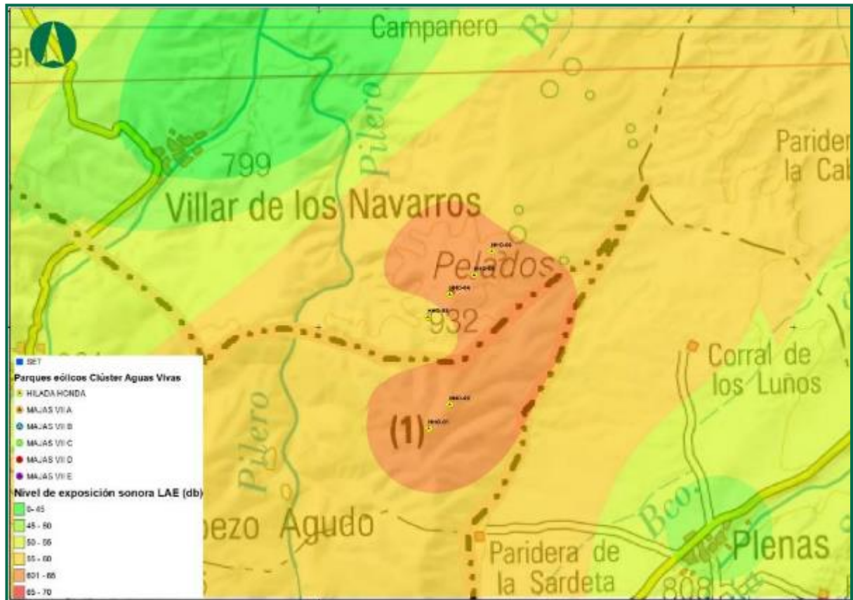
Figura 45. Distribución espacial hallada mediante dos tipos de interpolación diferentes (IDW) de los datos medidos en campo con una velocidad de viento entre 5 y 8 m/s y parques eólicos en funcionamiento.
