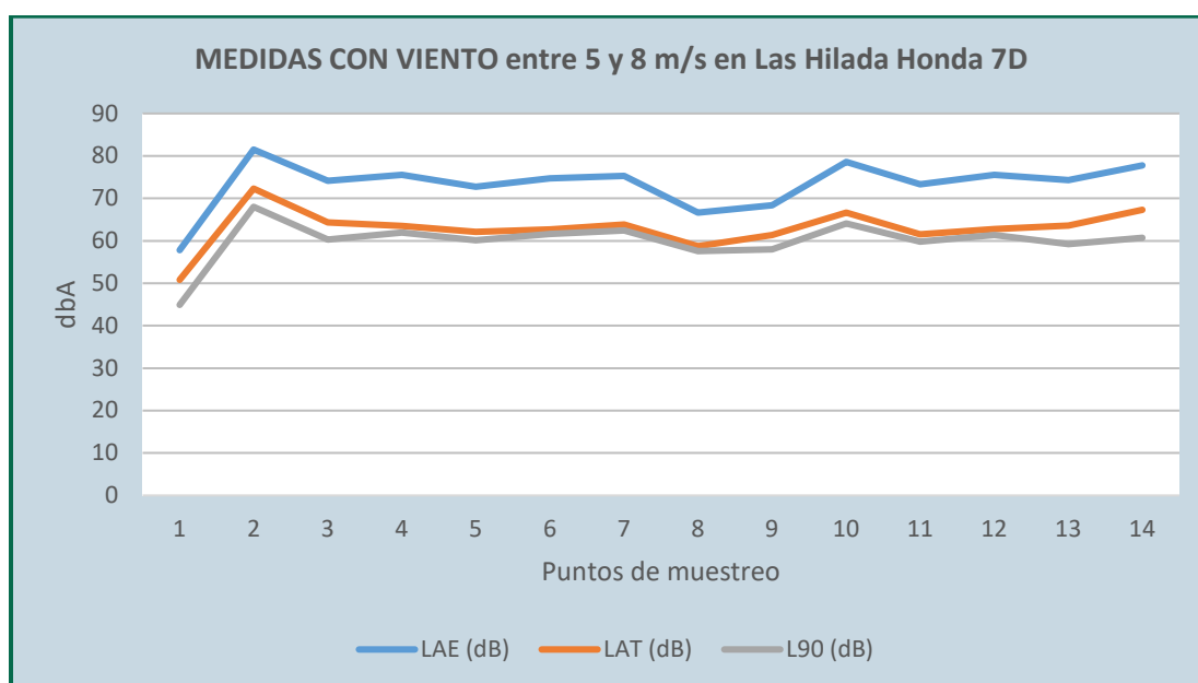
Figura 44. Registros en los puntos de medida., entre 5 y 8 m/s
