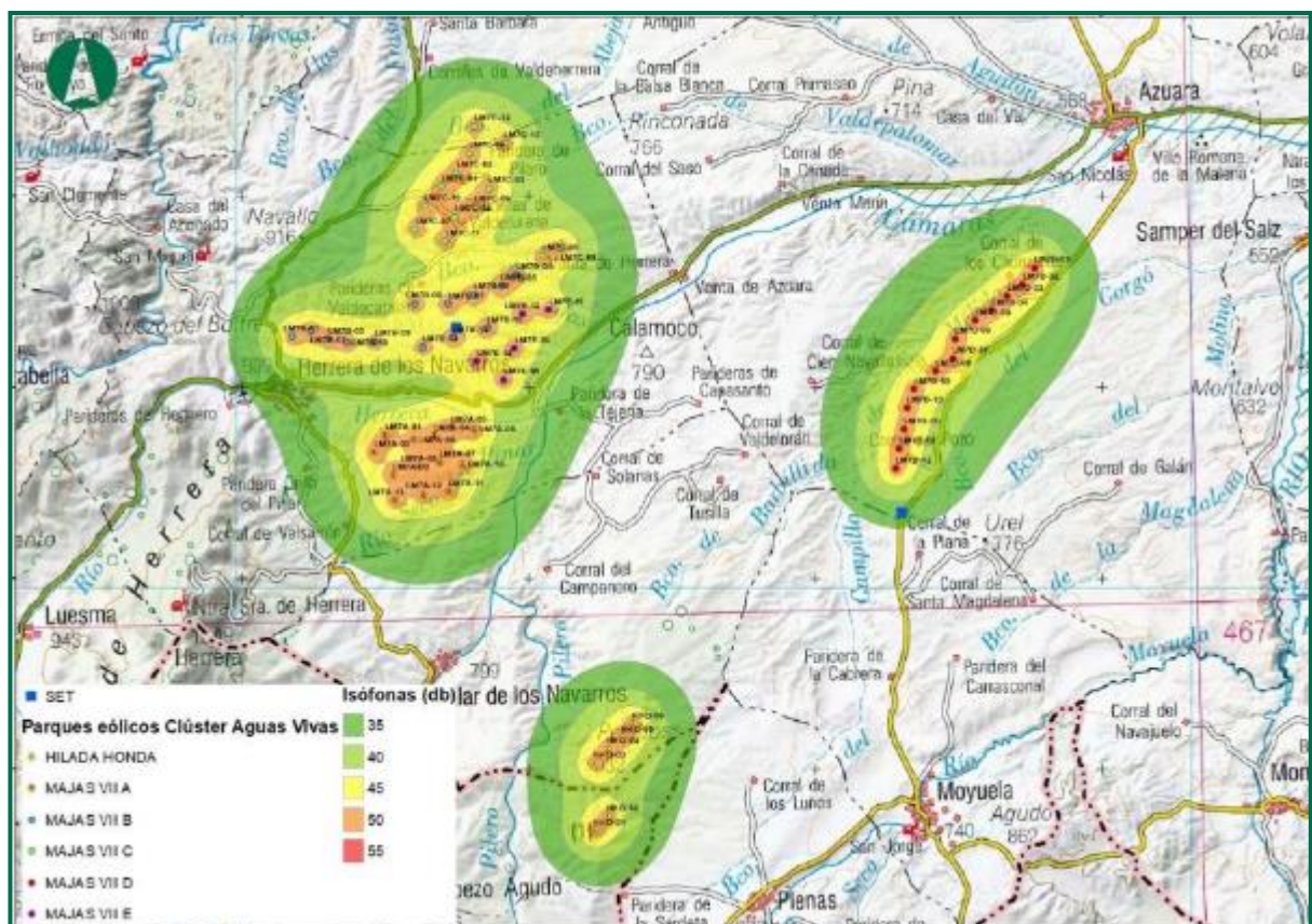
Figura 43. Niveles de presión sonora obtenidos.
