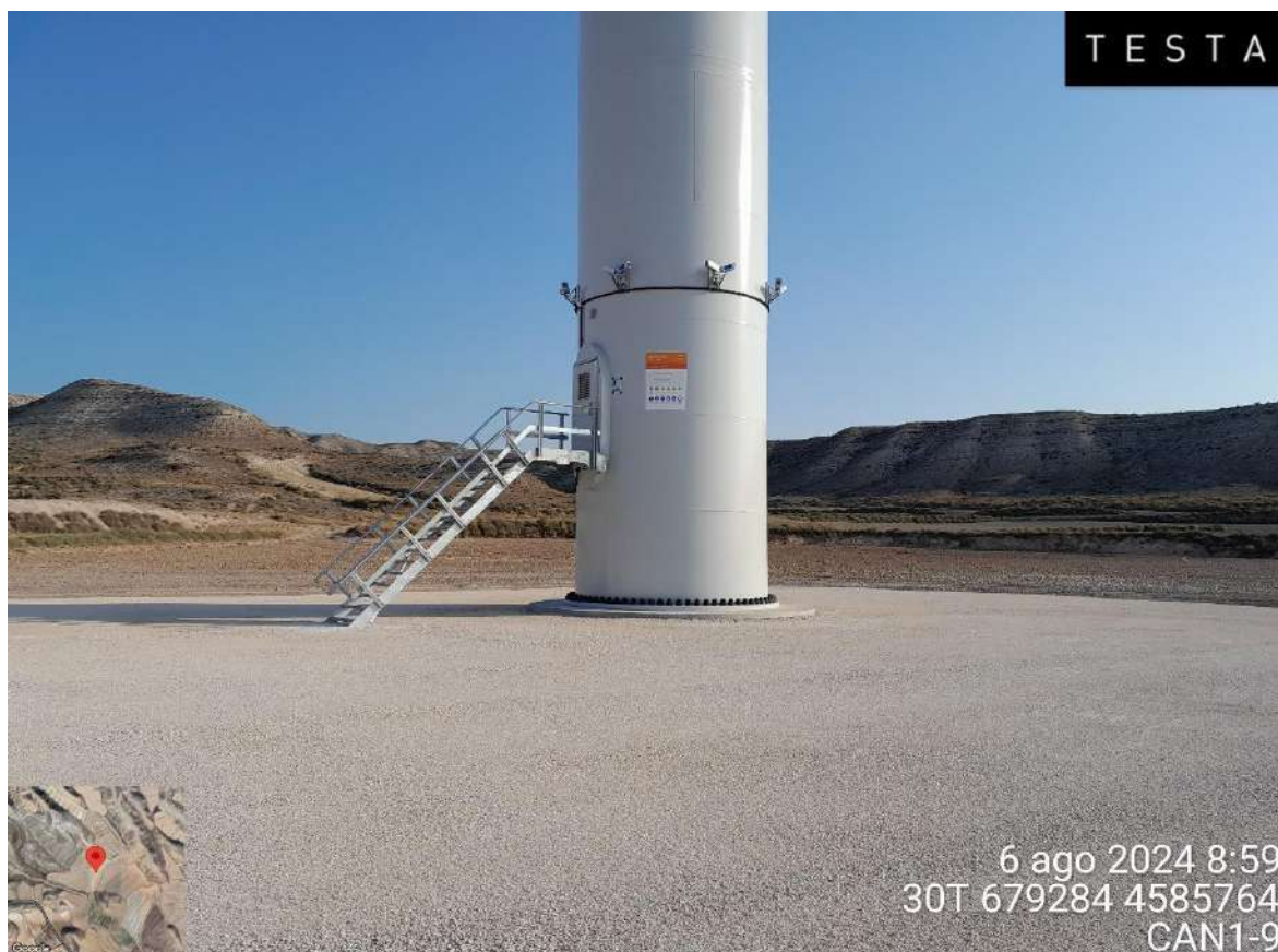
Imagen 2. Plataforma CAN1-09 y sistema de detección de avifauna
