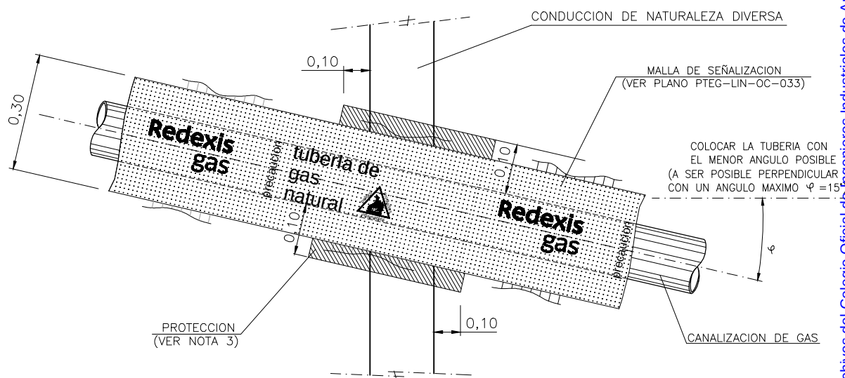
PLANTA
